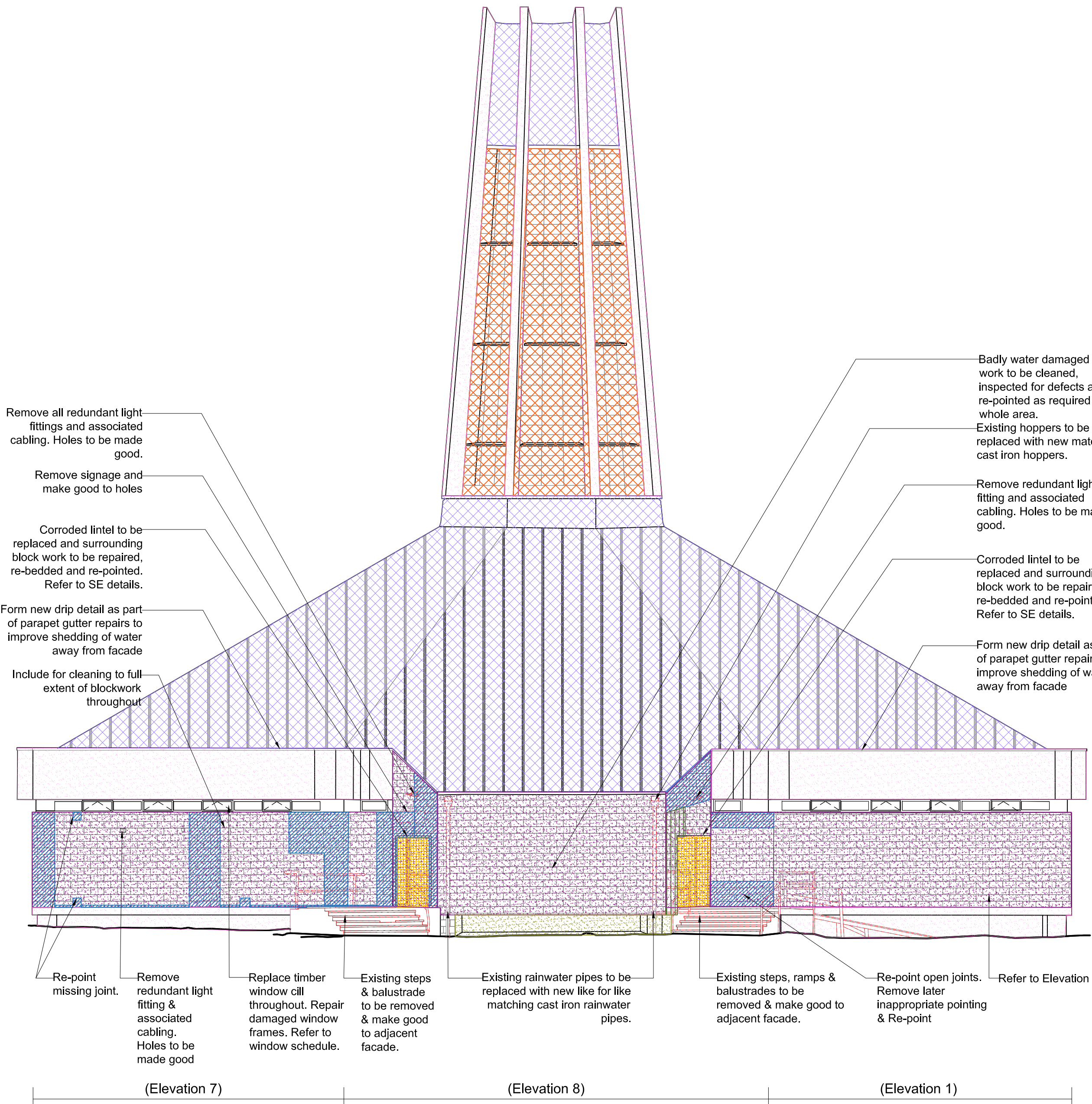
Elevation A
