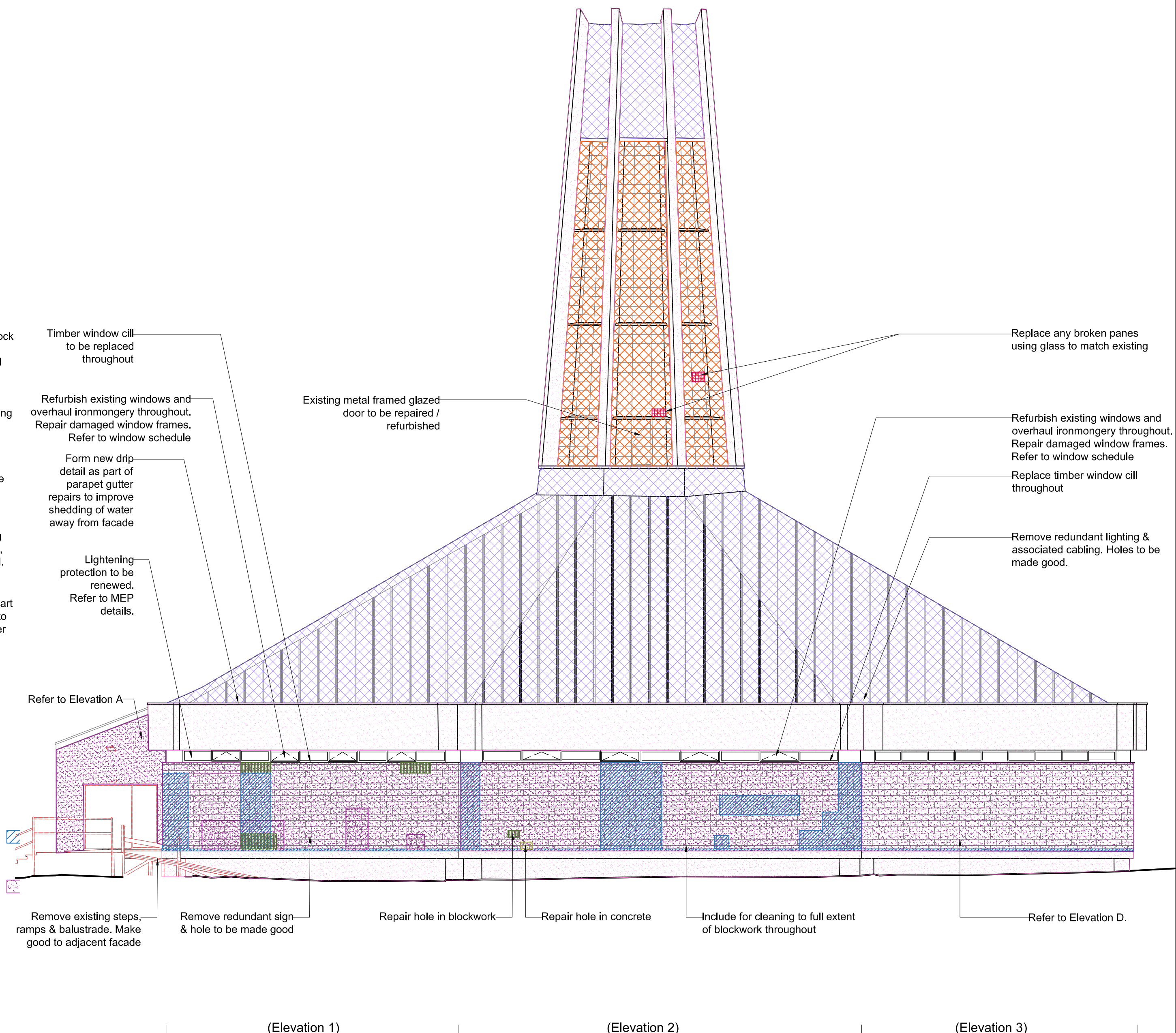
Elevation B
