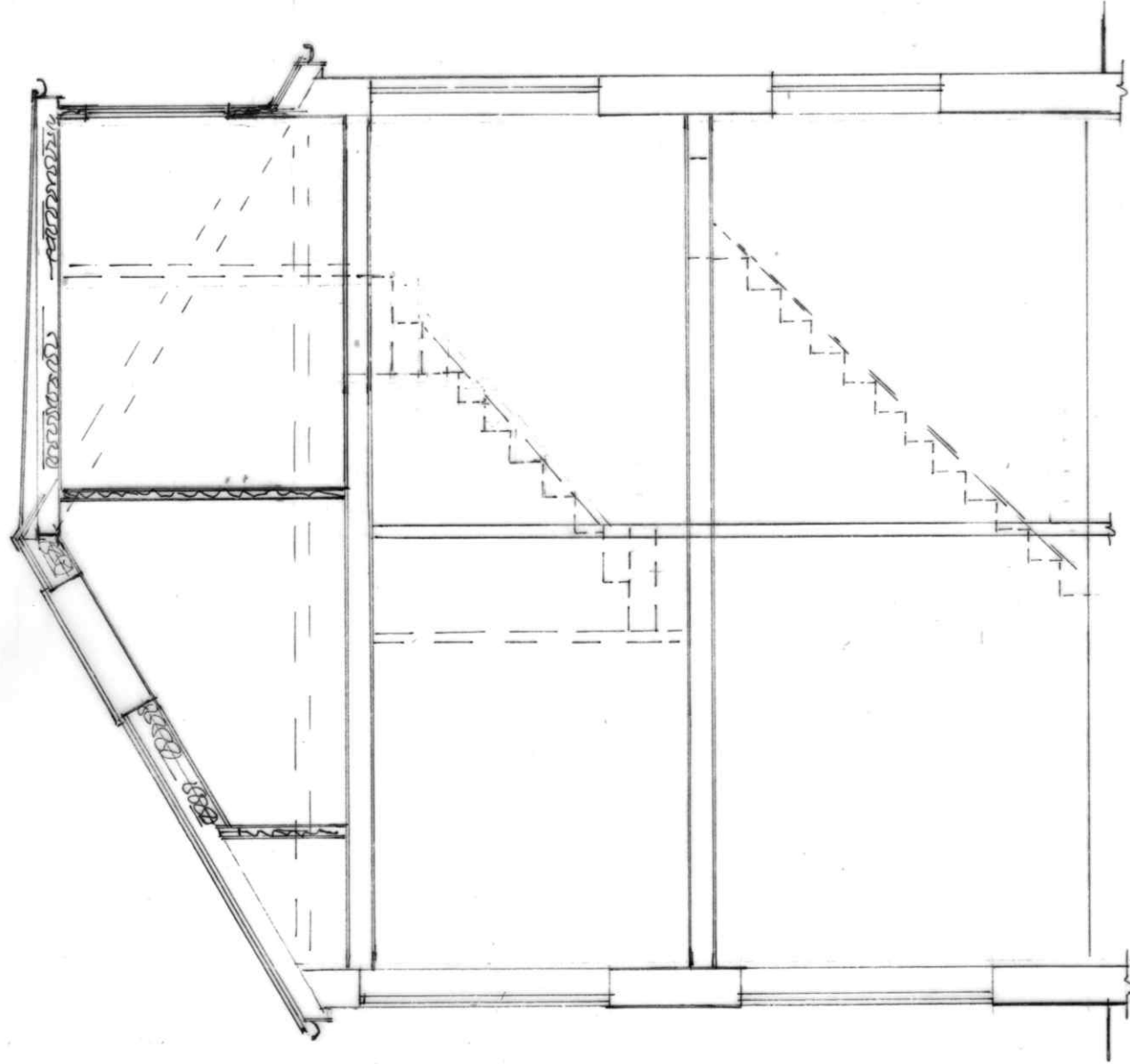
SECTION A.A
