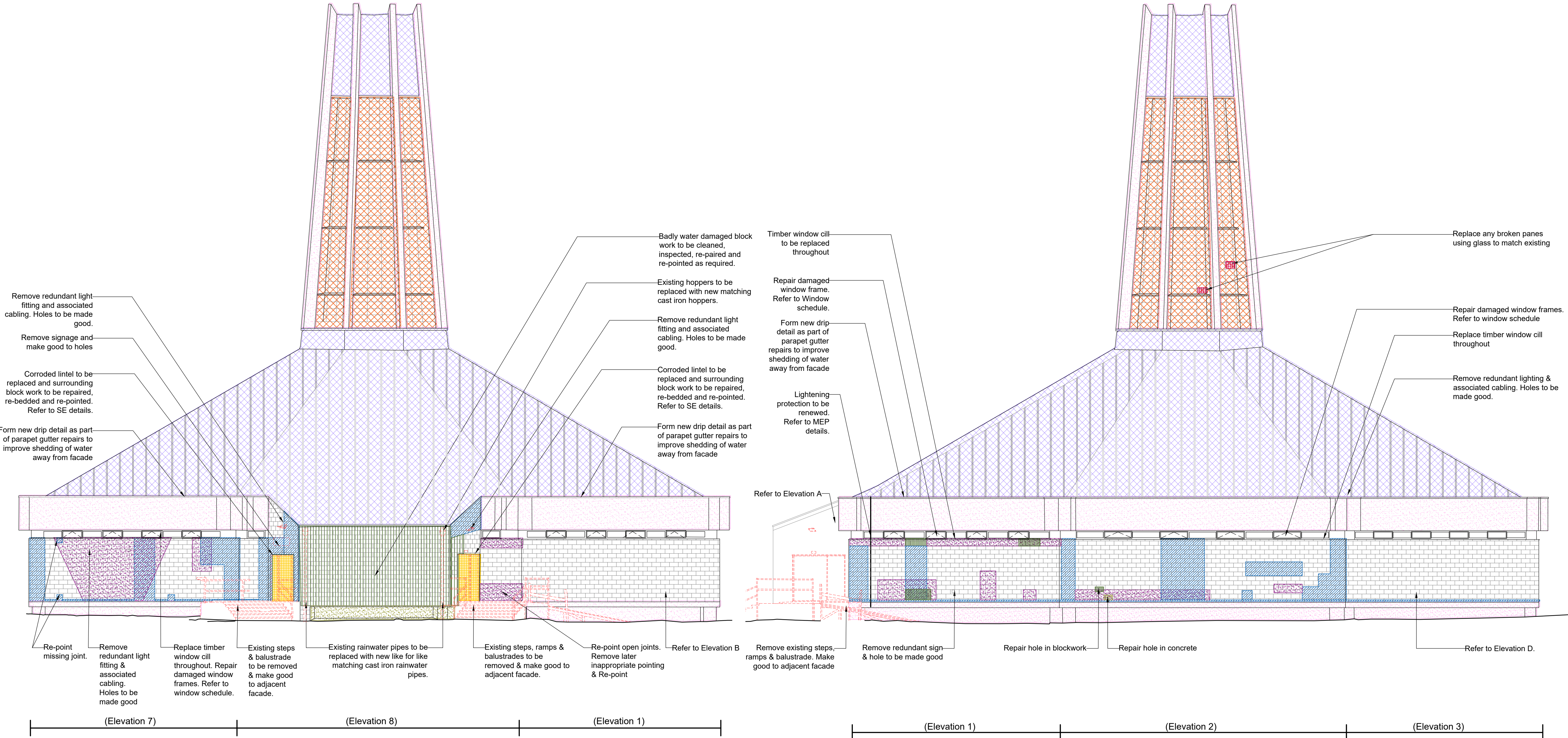
Elevation A
