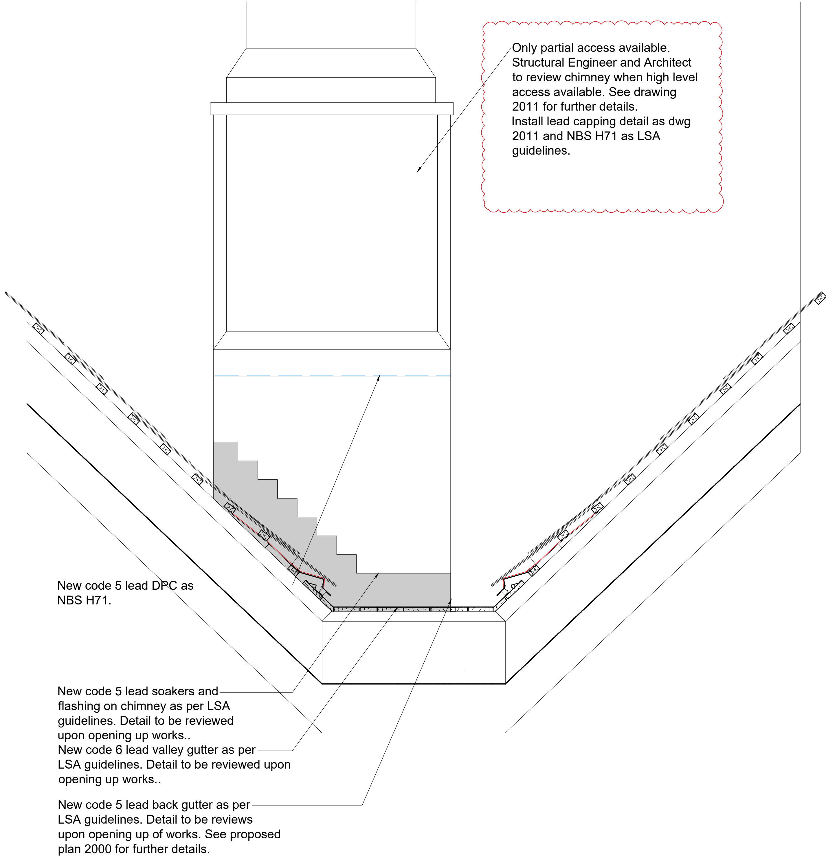
02 - Chimney
