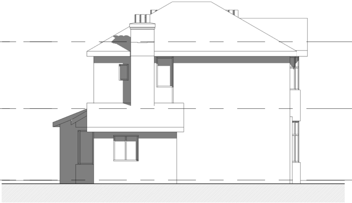
2 Left Side - Existing 1 : 100
