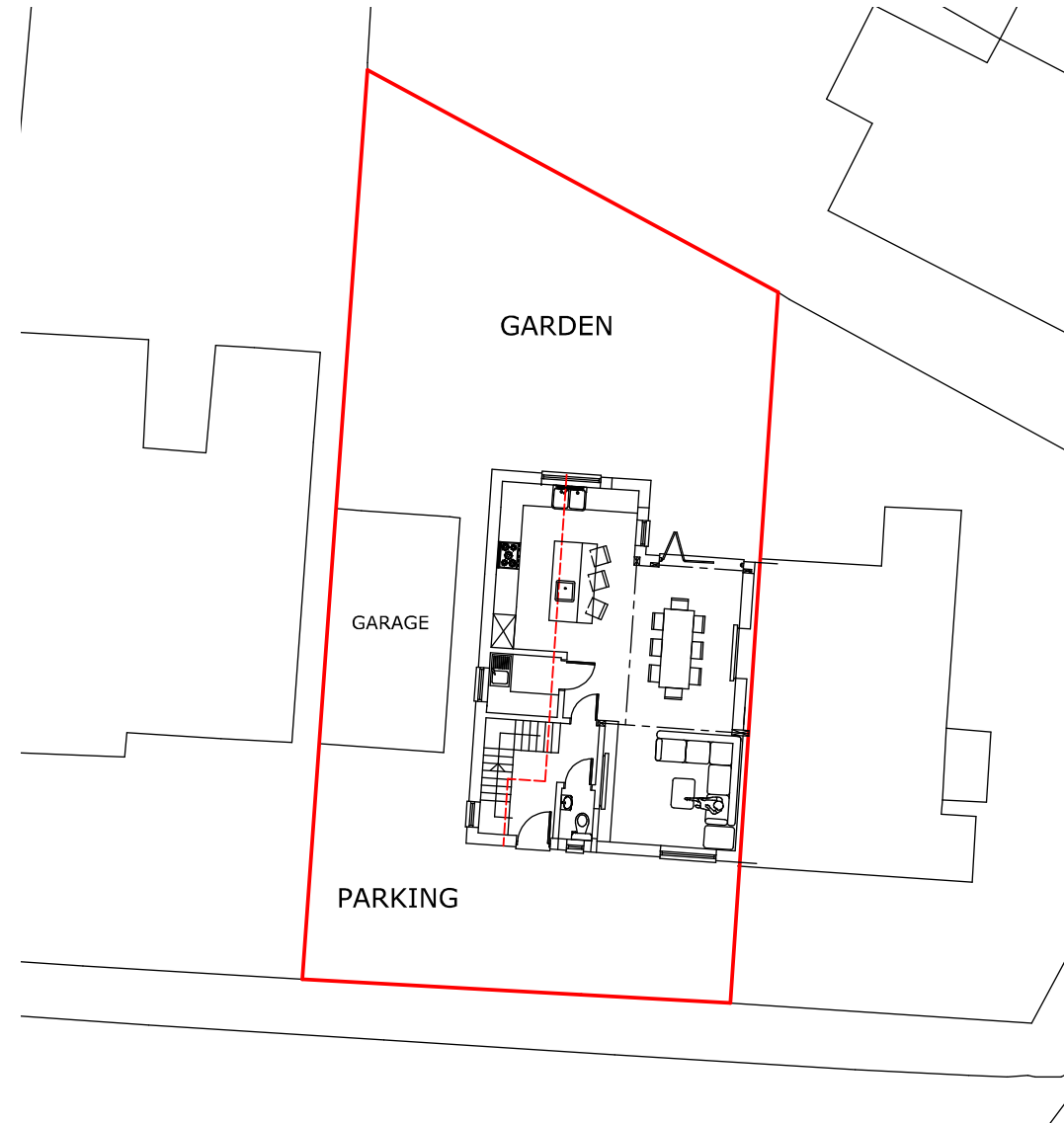
site plan 1:200
