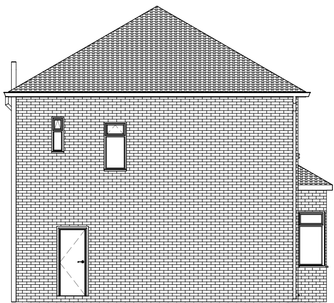
Existing Side 1 : 100
