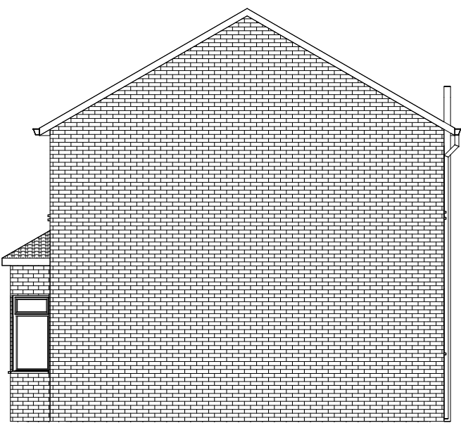
Existing Side (2) 1 : 100
