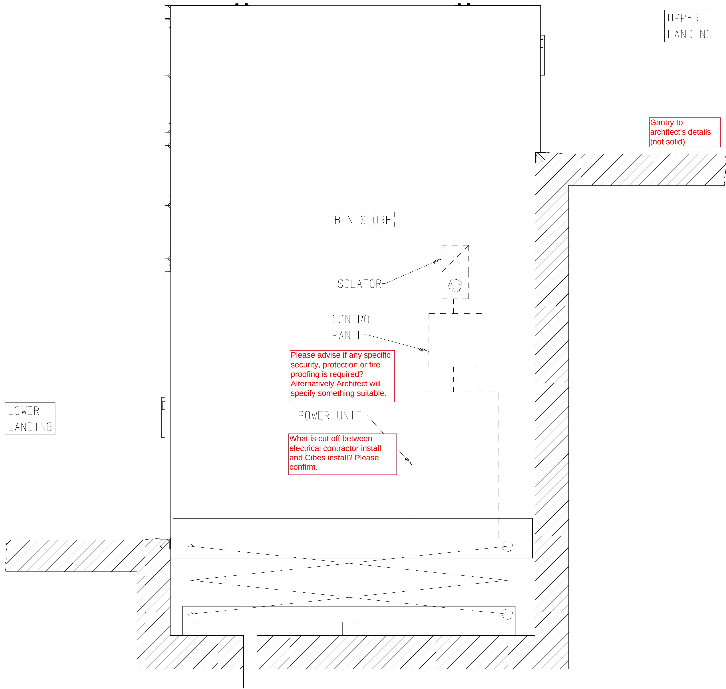
SECTION A-A
