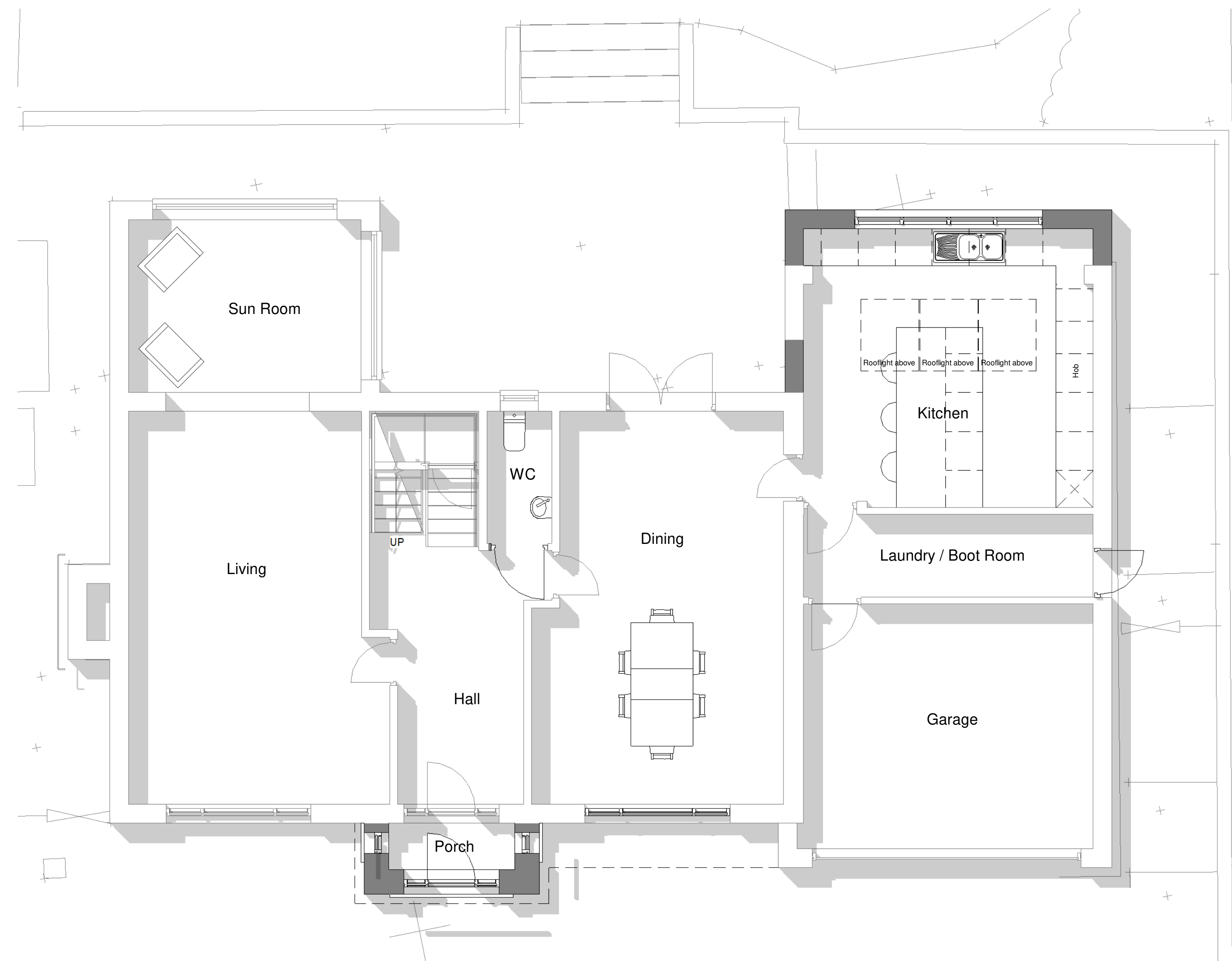
1 | PRO Level 0 1 : 50
