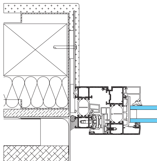
Jamb detail
