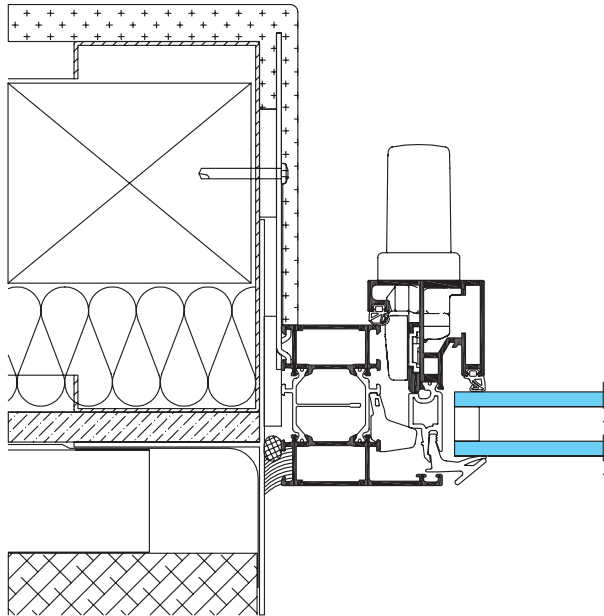
Jamb detail
