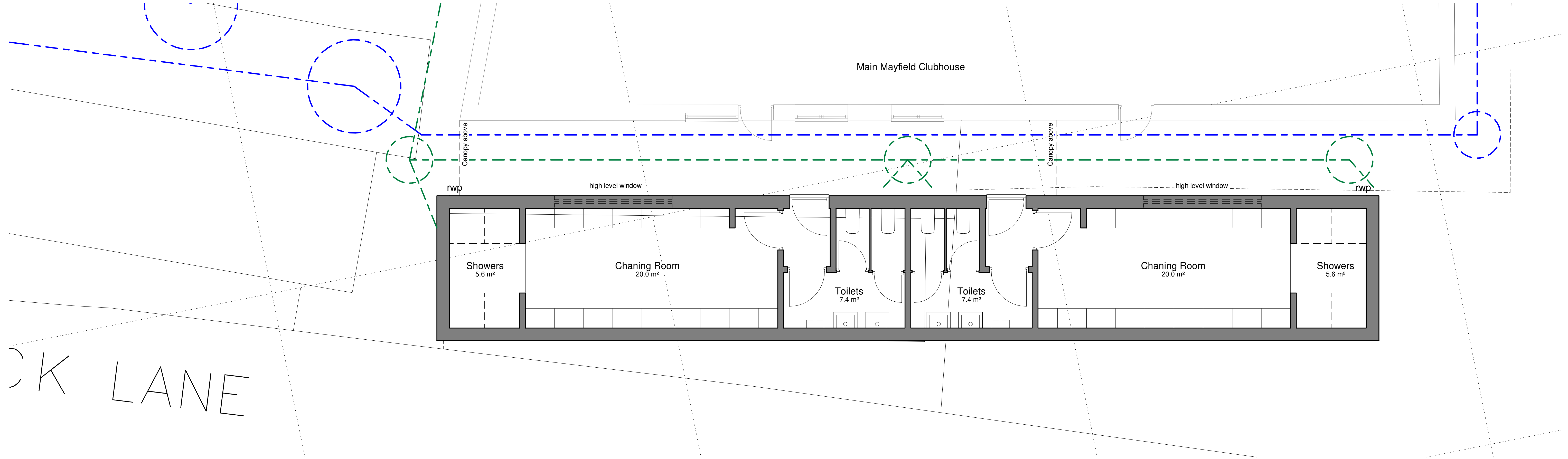
2 | Pro Level 0 1 : 50
