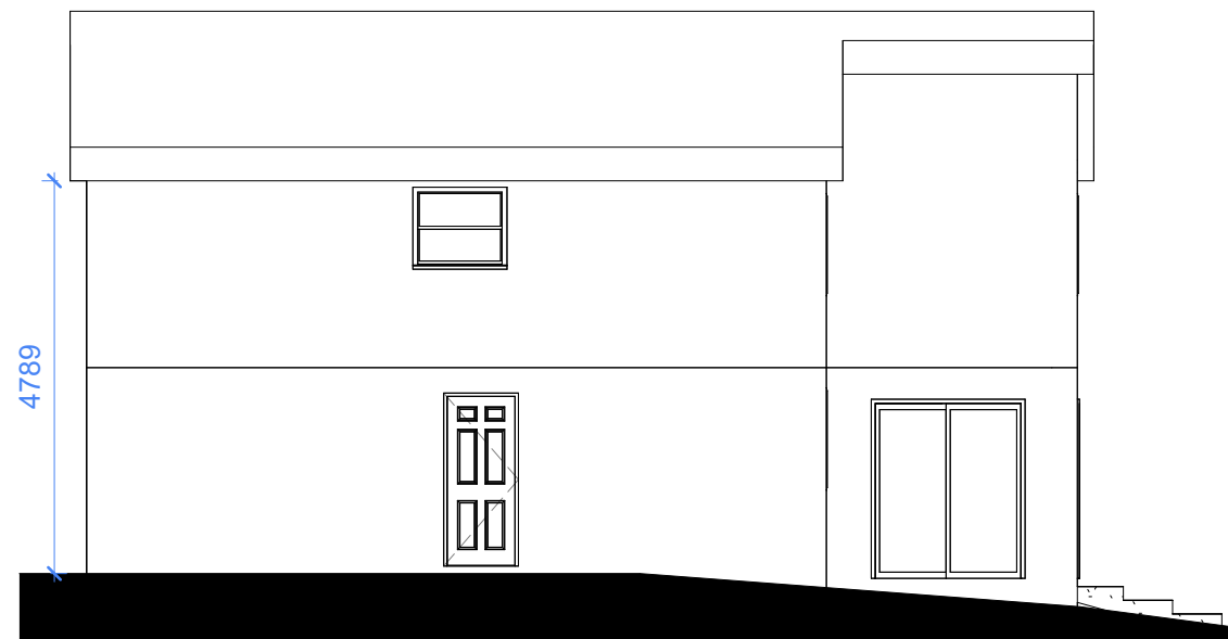
West - Side 1 : 100
