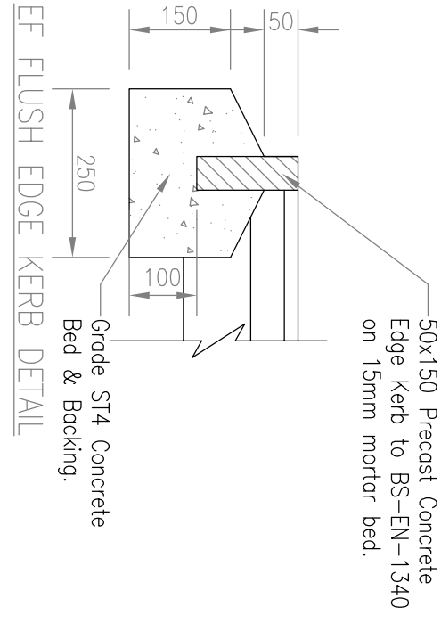
EF EDGE KERB DETAIL
