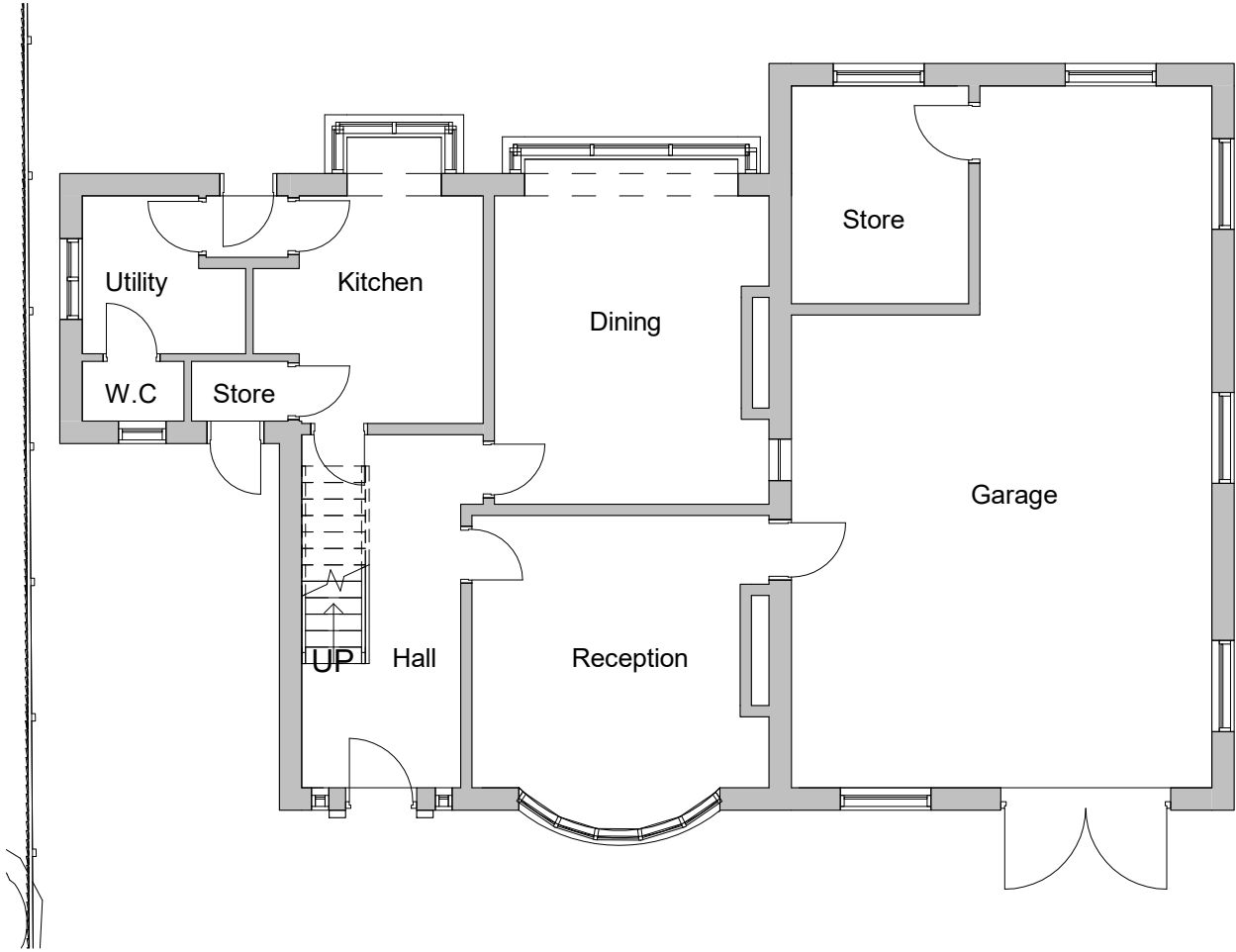
1 Level 0 - Existing 1 : 100
