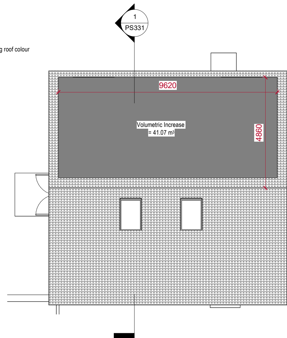
3 Roof Plan 1 : 100
