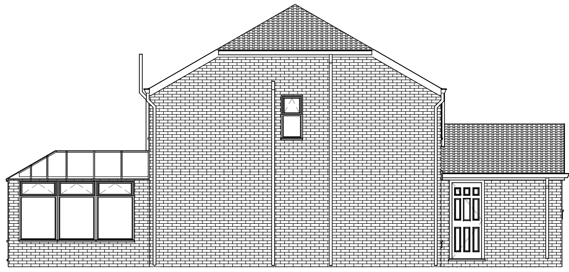
Existing Side II 1 : 100
