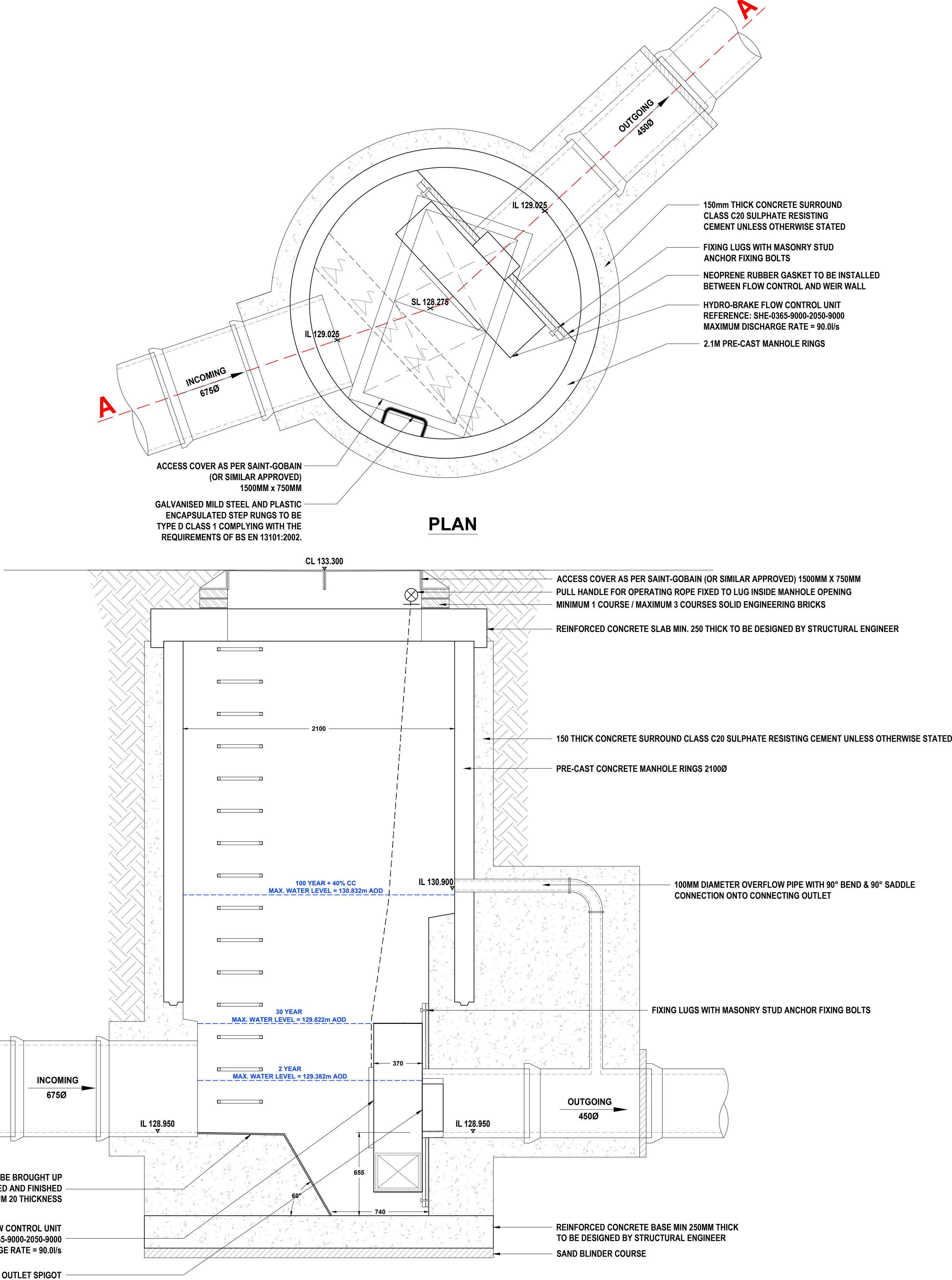
SECTION A-A
