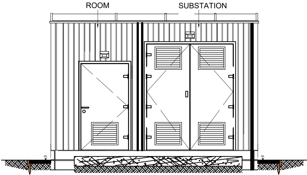
ELEVATION A
