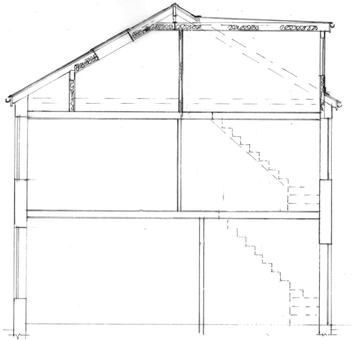
SECTION A.A
