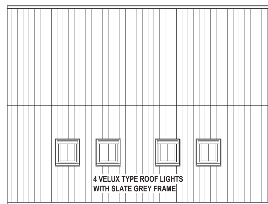
4 ROOF PLAN 1 : 100
