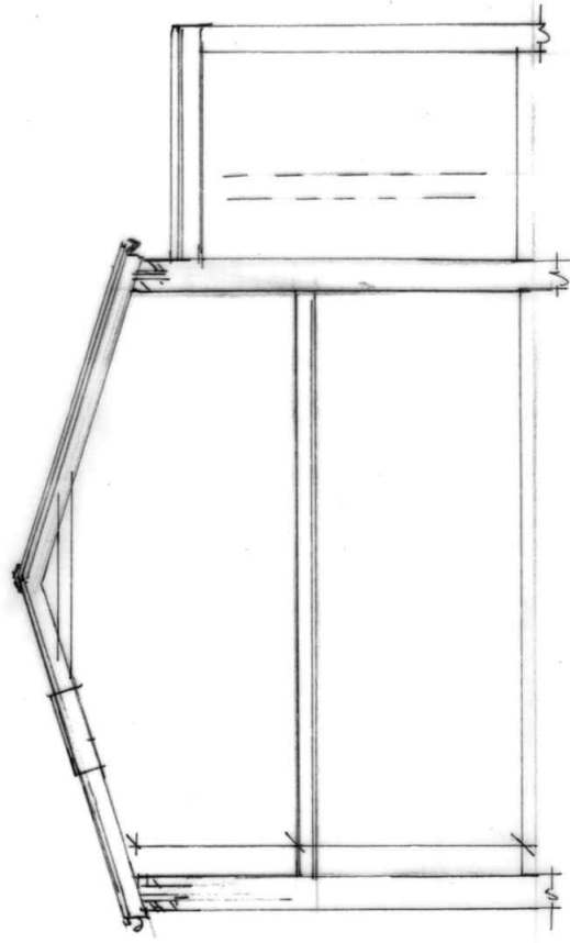
SECTION A.A
