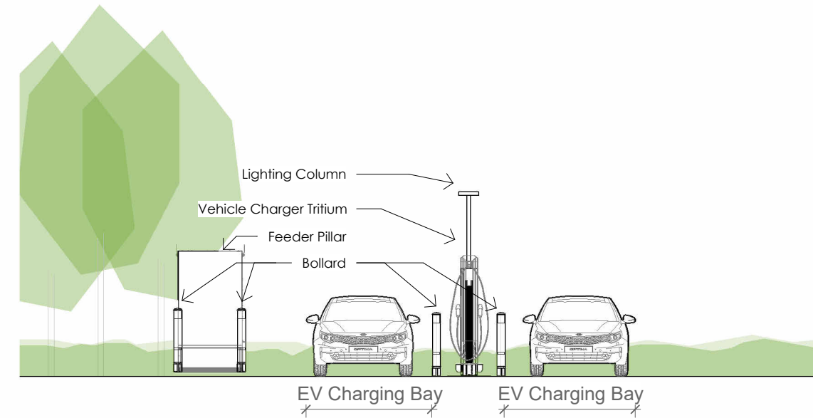
Section 4 1 : 100
