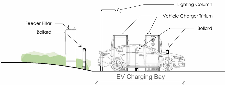
Section 2 1 : 100
