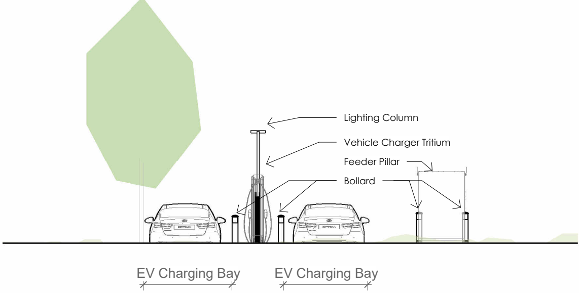
Section 3 1 : 100
