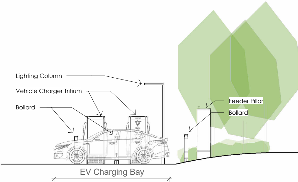
Section 1 1 : 100
