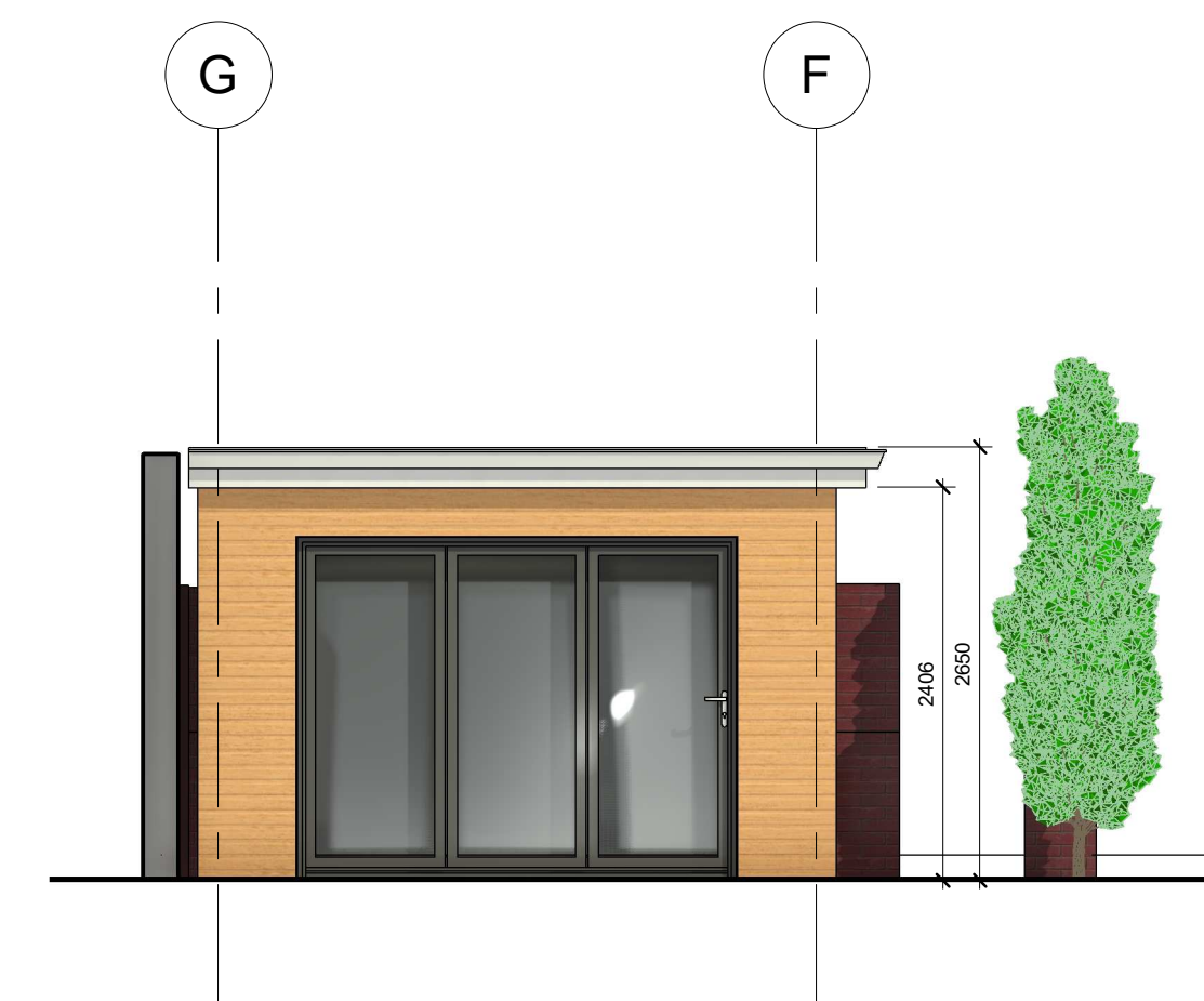
3 Elevation 2 - a 1 : 50
