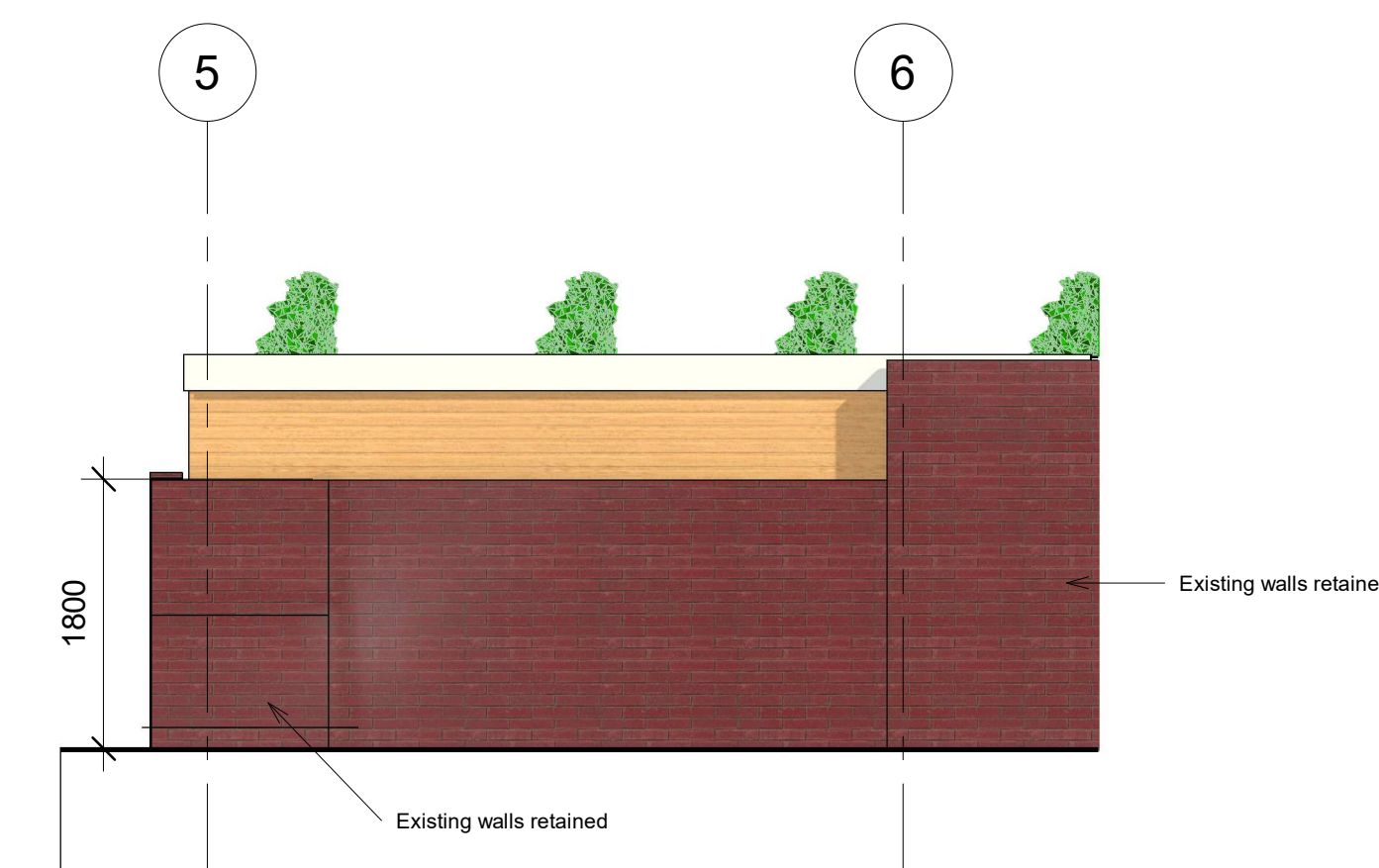
4 Elevation 3 - a 1 : 50
