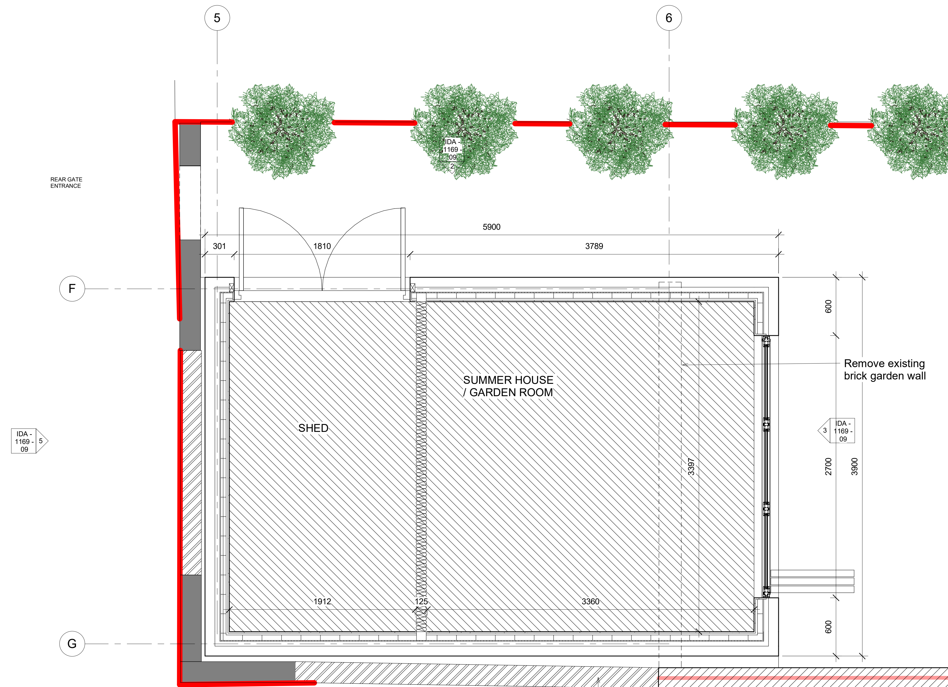
1 Garden room plan 1 : 20
