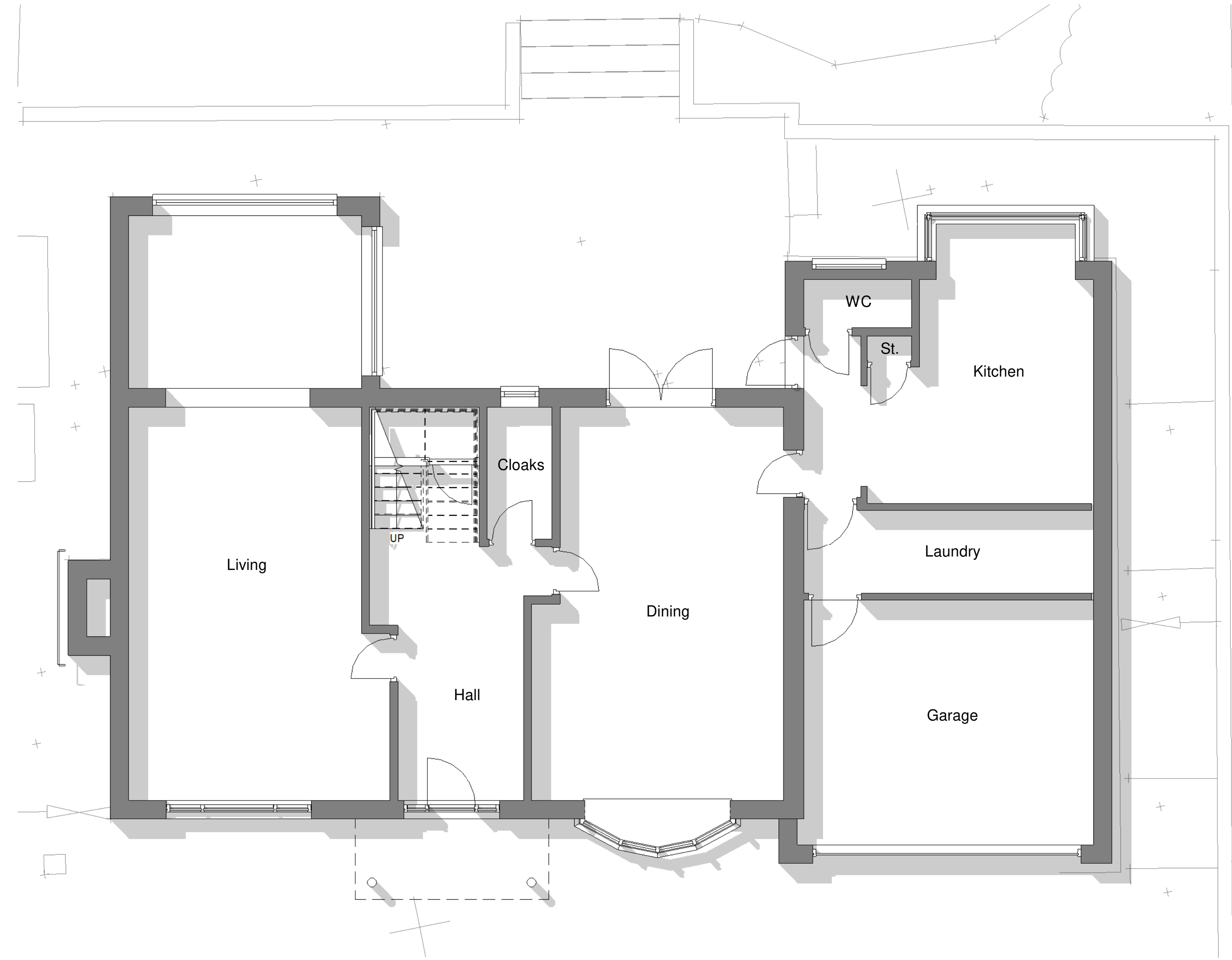
1 | Ex Level 0 1 : 50
