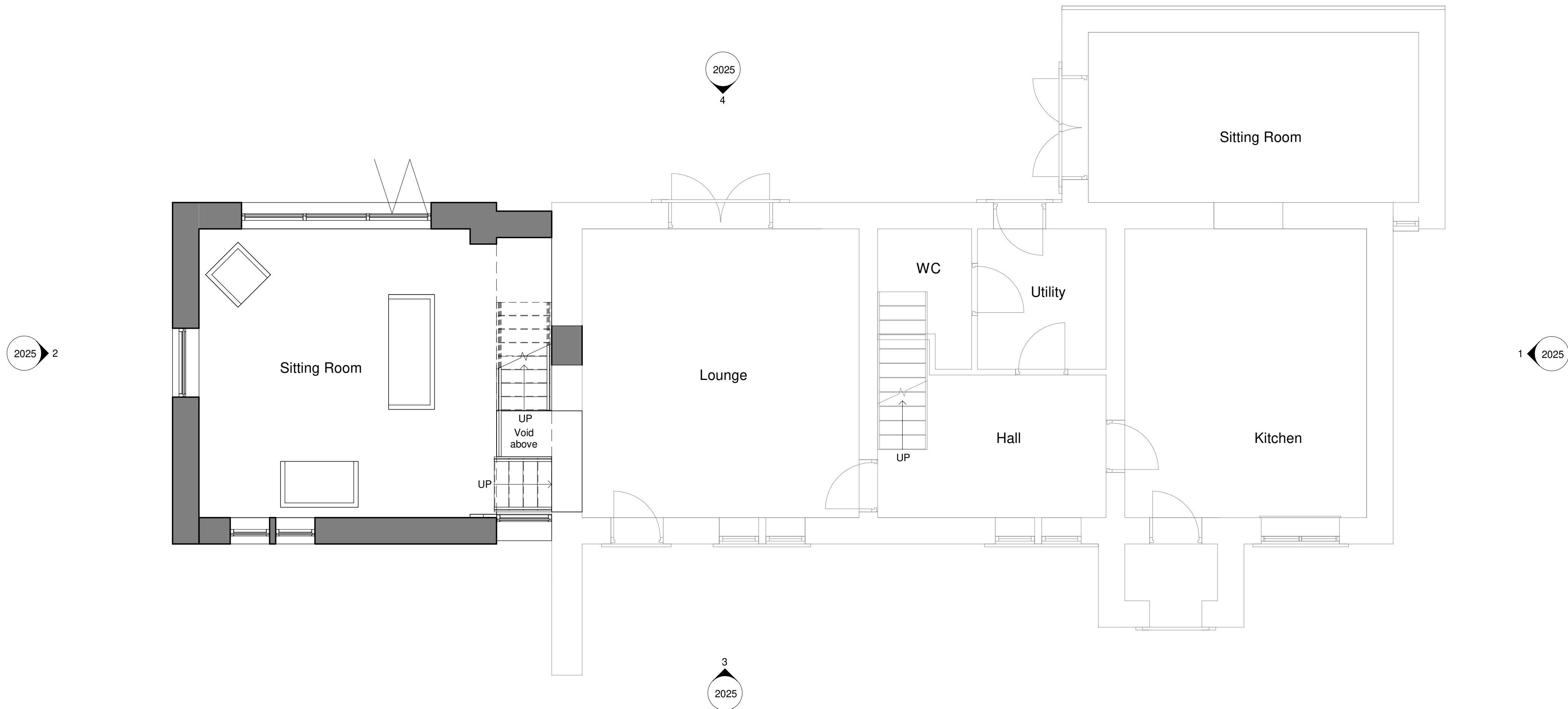
1 | Pro Level 0 1 : 50
