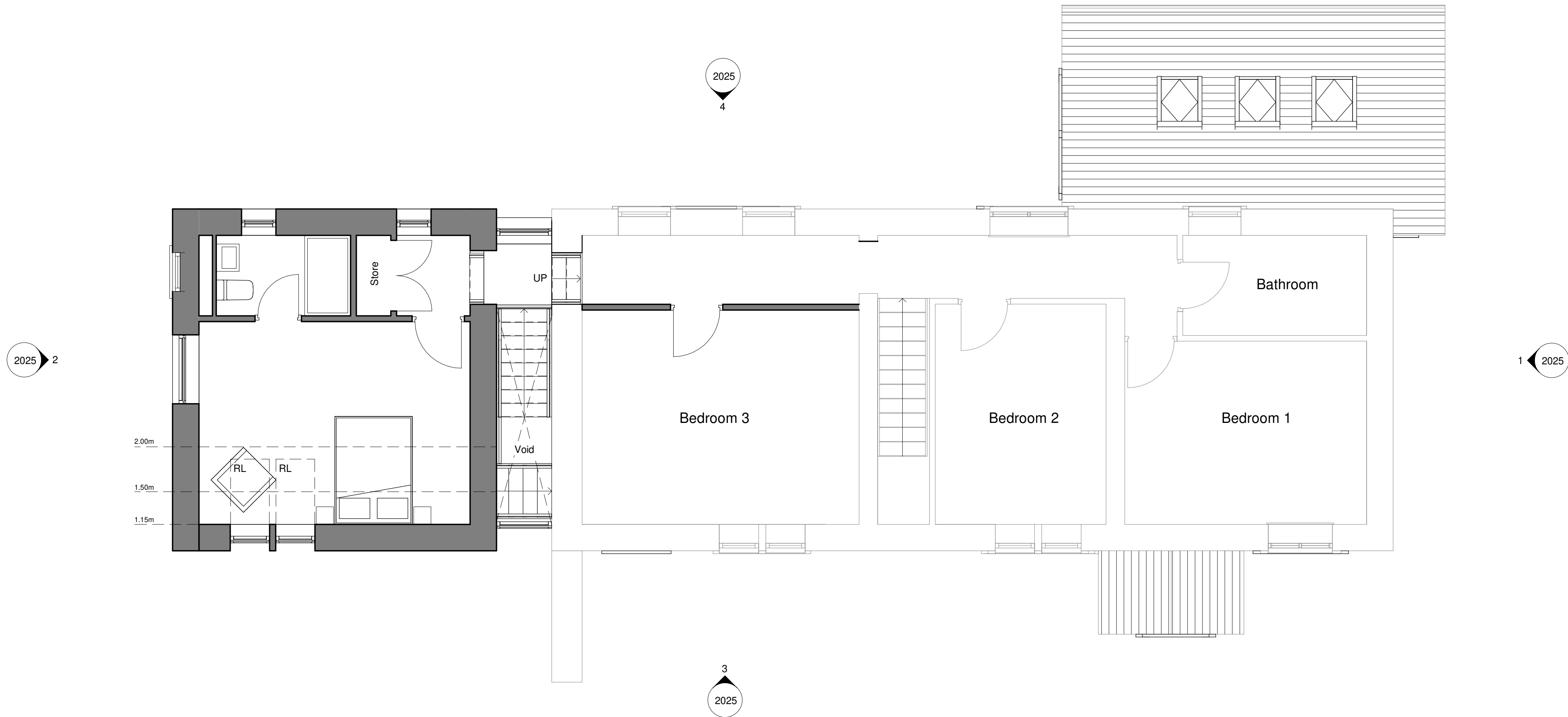
2 | Pro Level 1 1 : 50
