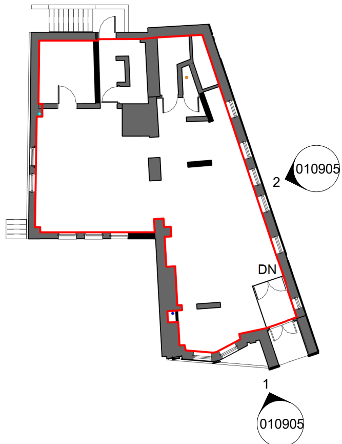
KEY PLAN 1 : 200
