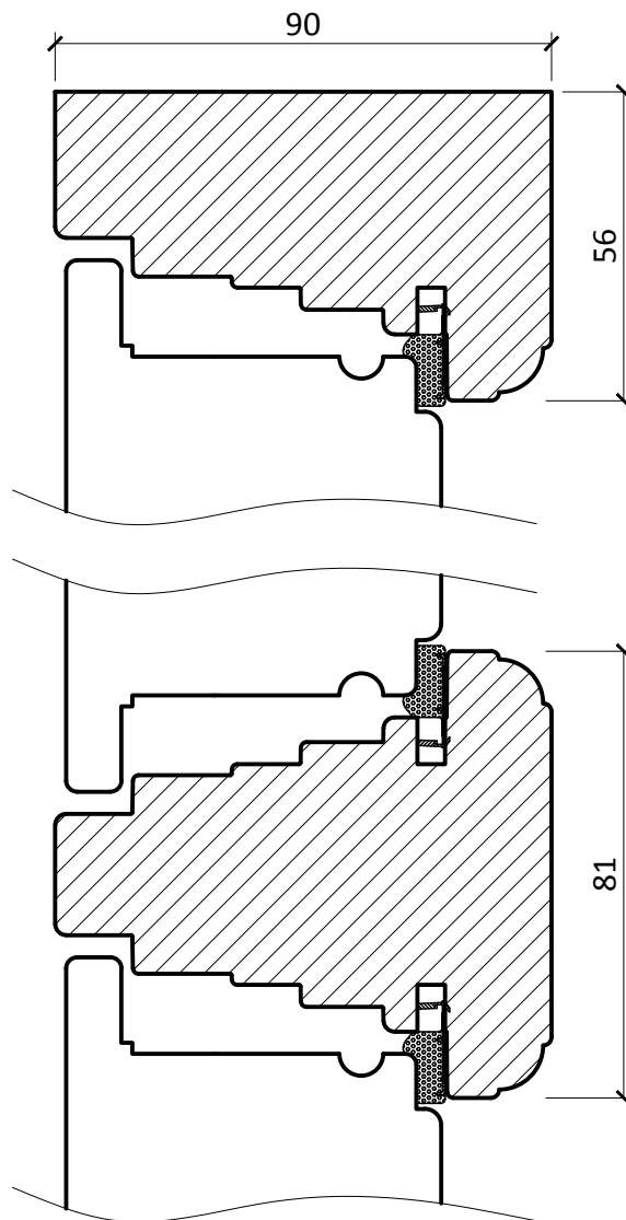
Ovolo frame
