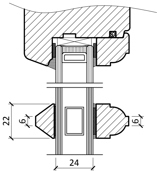
Ovolo Profile 1
