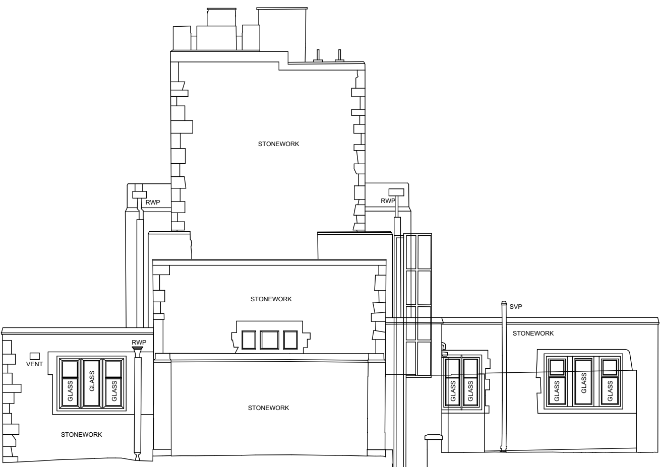
Datum 134.00m Elevation 2
