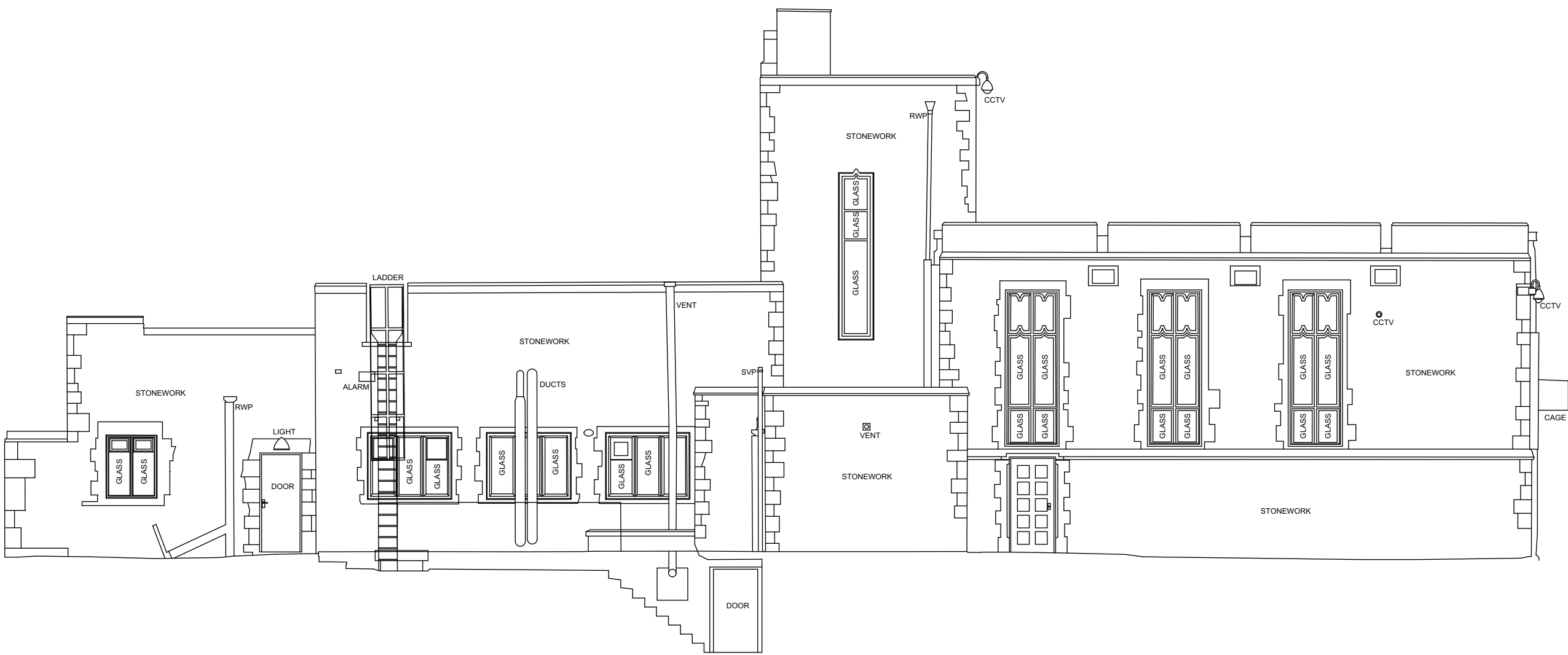
Datum 132.00m Elevation 3
