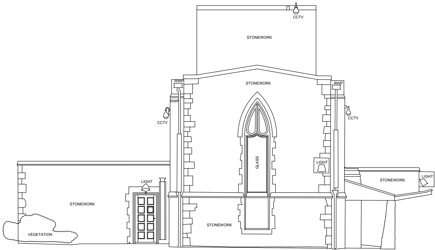
Datum 134.00m Elevation 4
