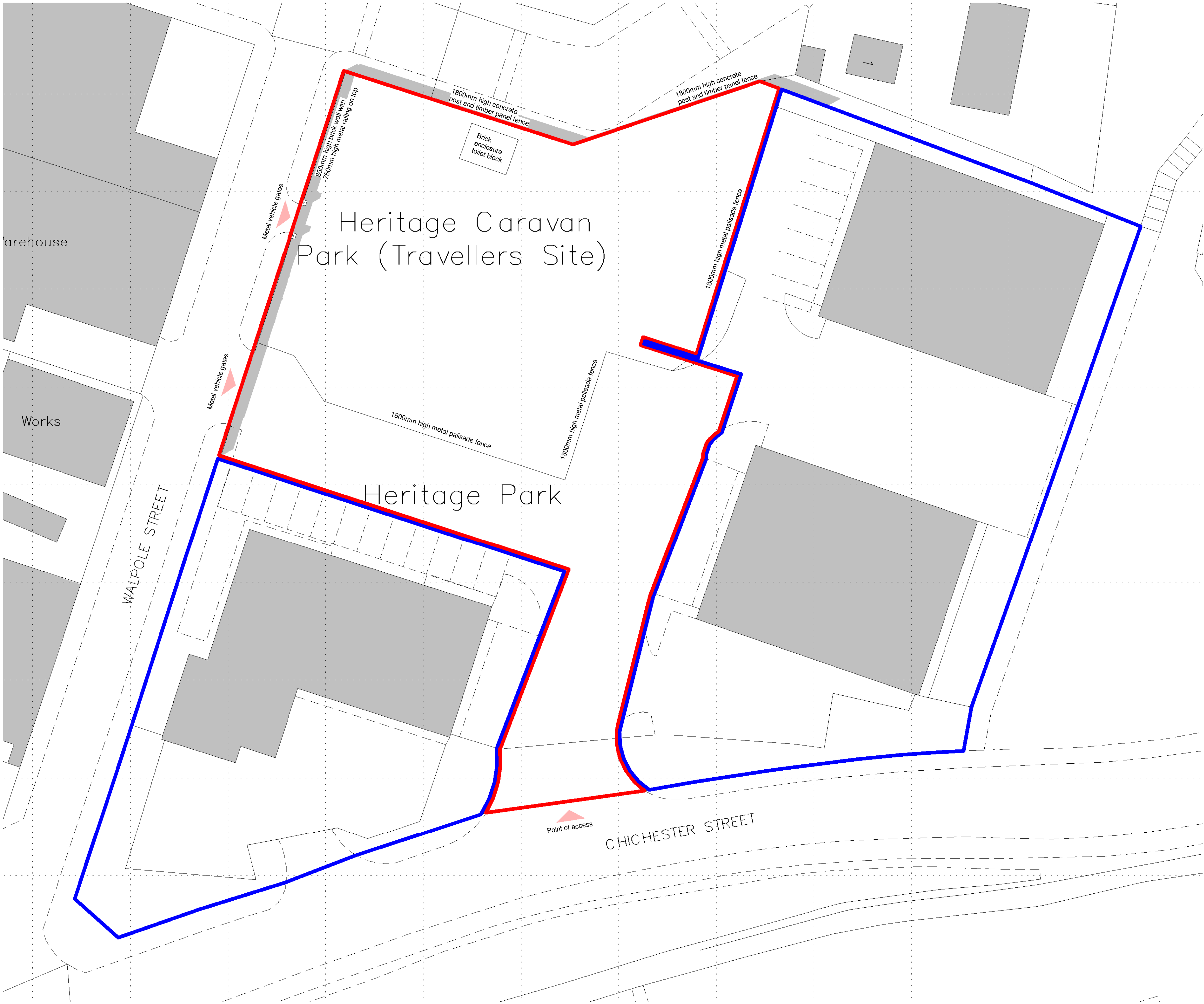
2 Ex Site Plan 1 : 200
