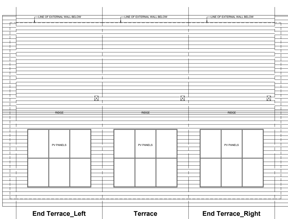
2 BED 3P - ROOF
