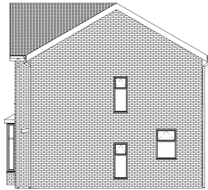
Existing Side (2) 1 : 100
