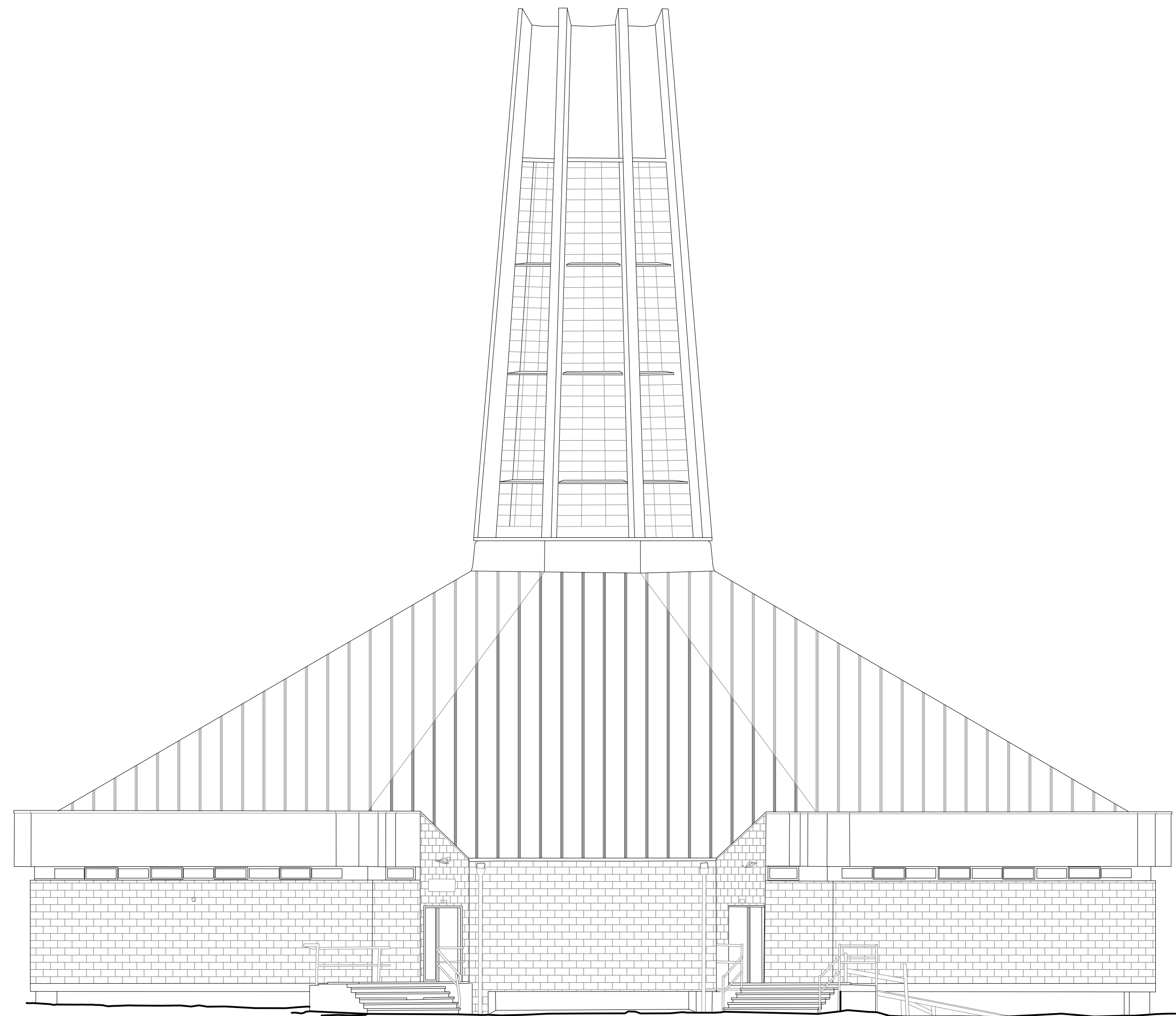
Elevation A
