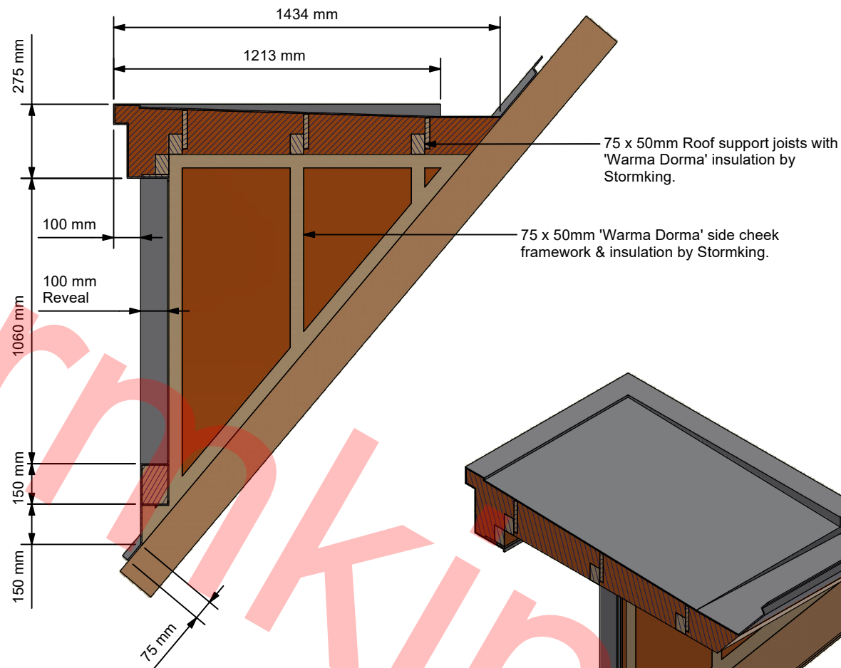
A-A ( 1:20 )
