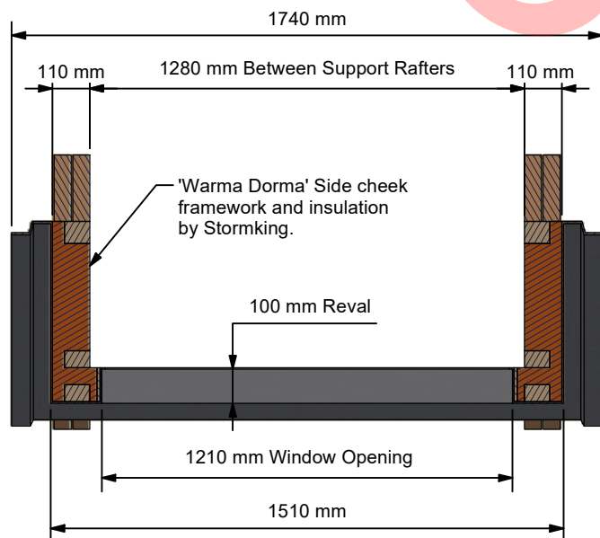
B-B ( 1:20 )
