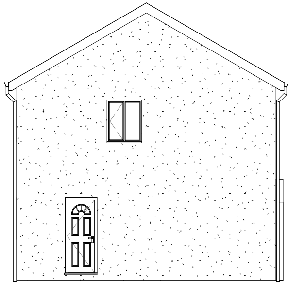
Existing Side 1 : 100
