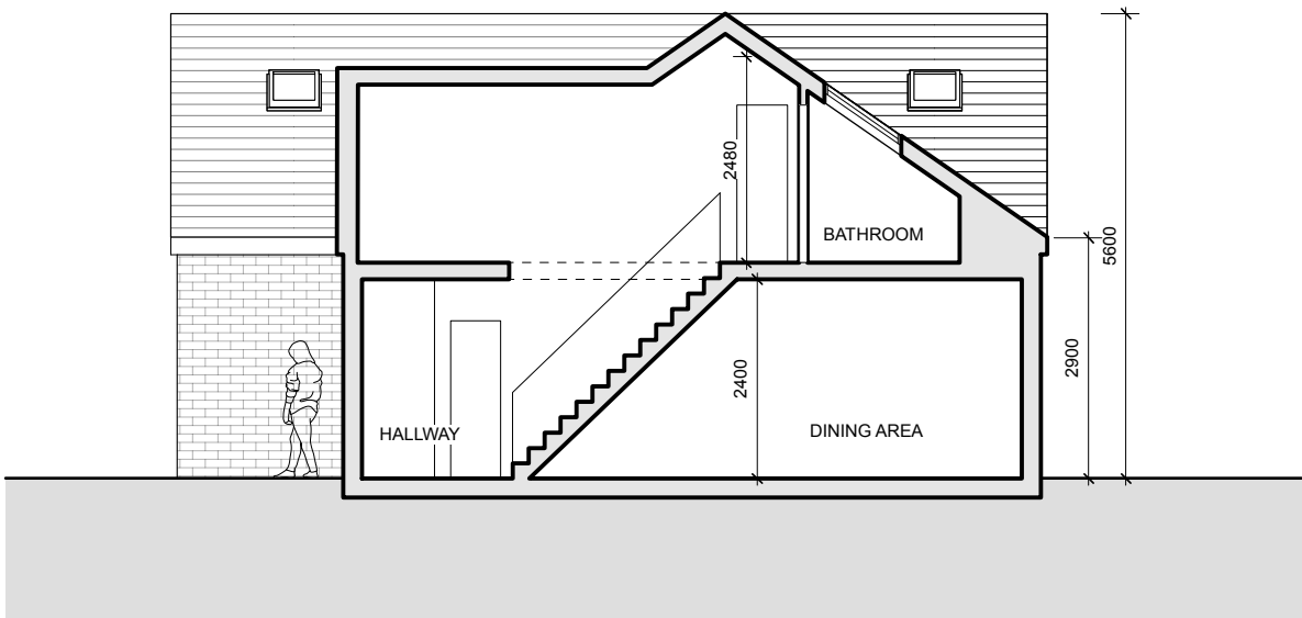
PROPOSEDSECTION B-B
