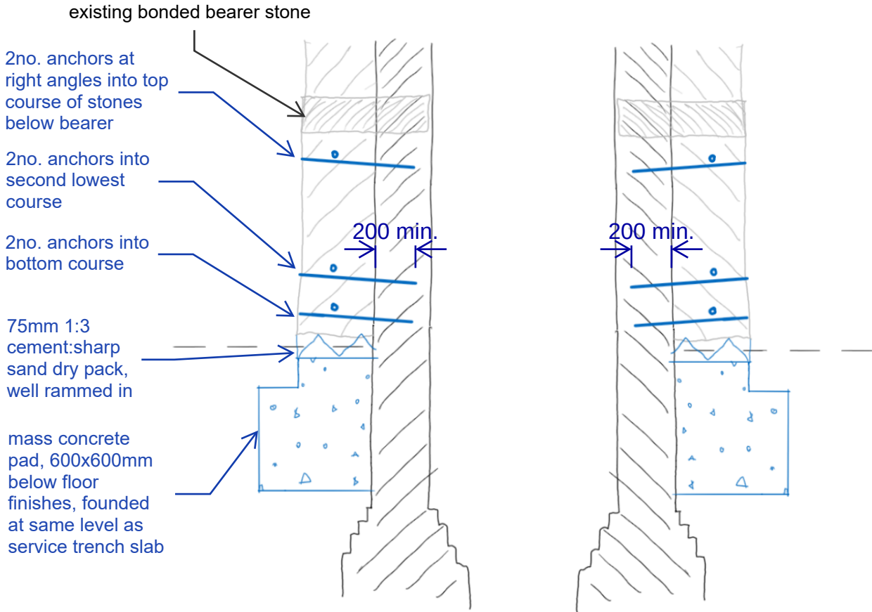
C-C
