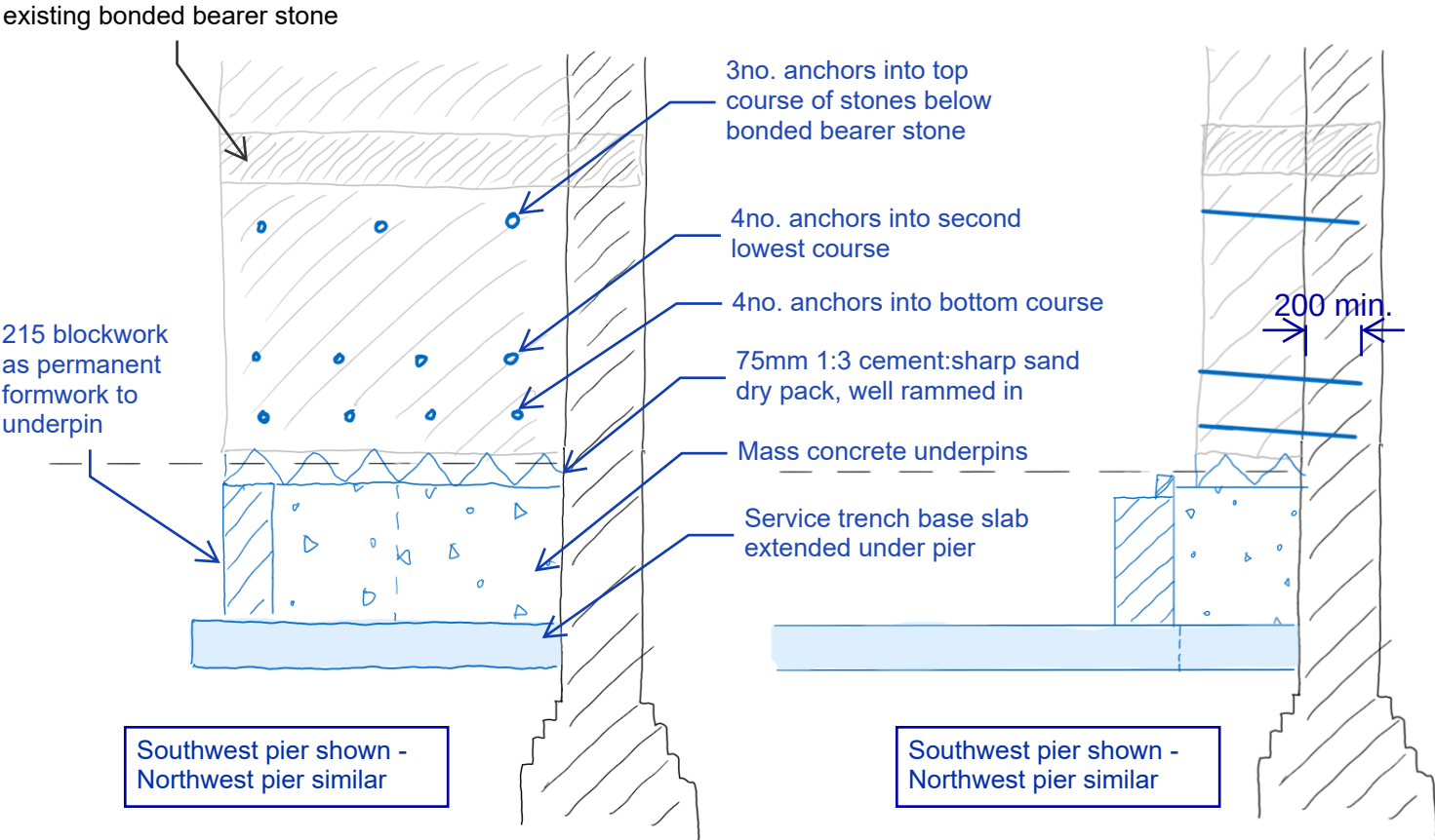
A-A
