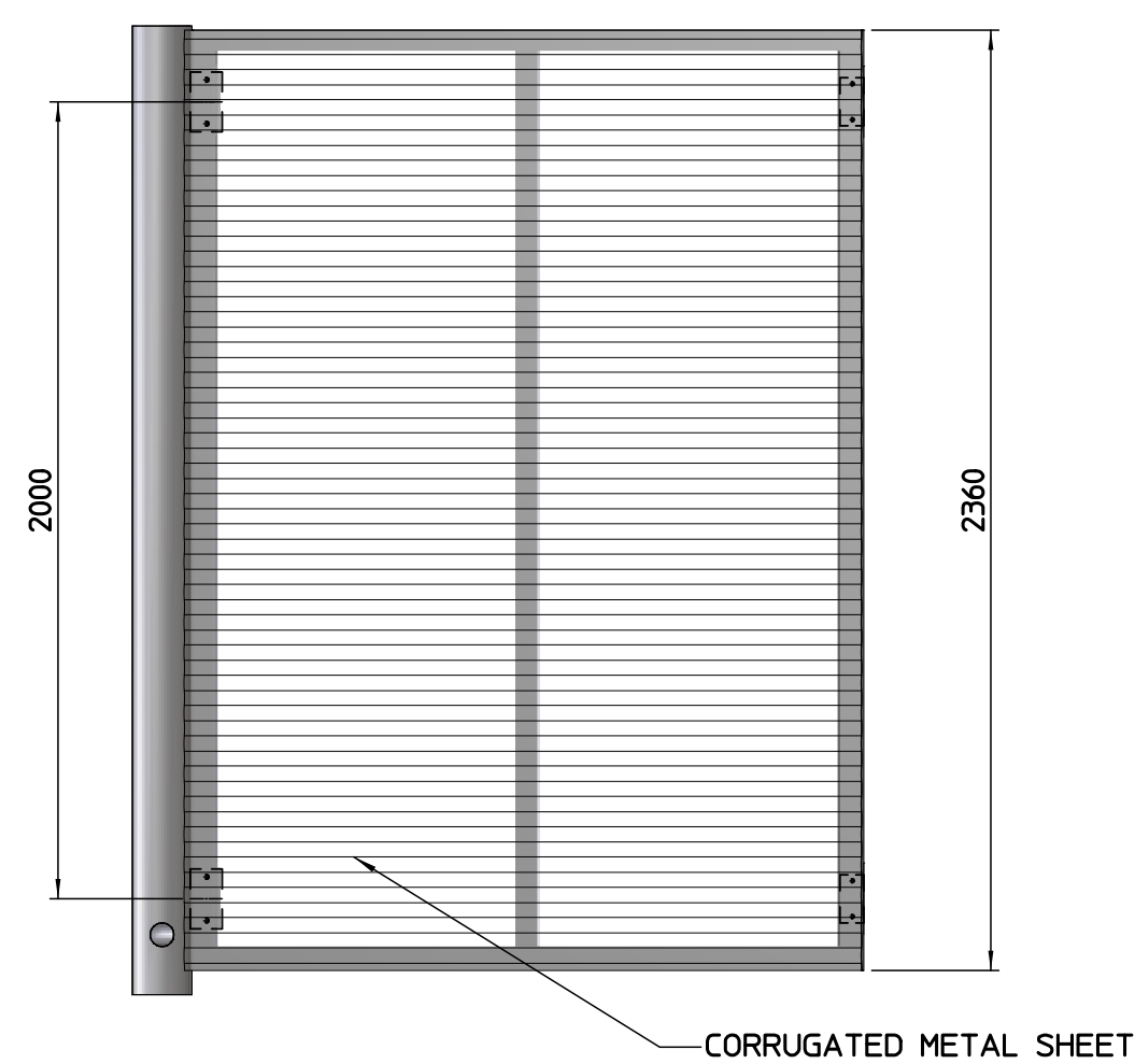
VISTA DALL'ALTO - top view1 SCALE 1:20
