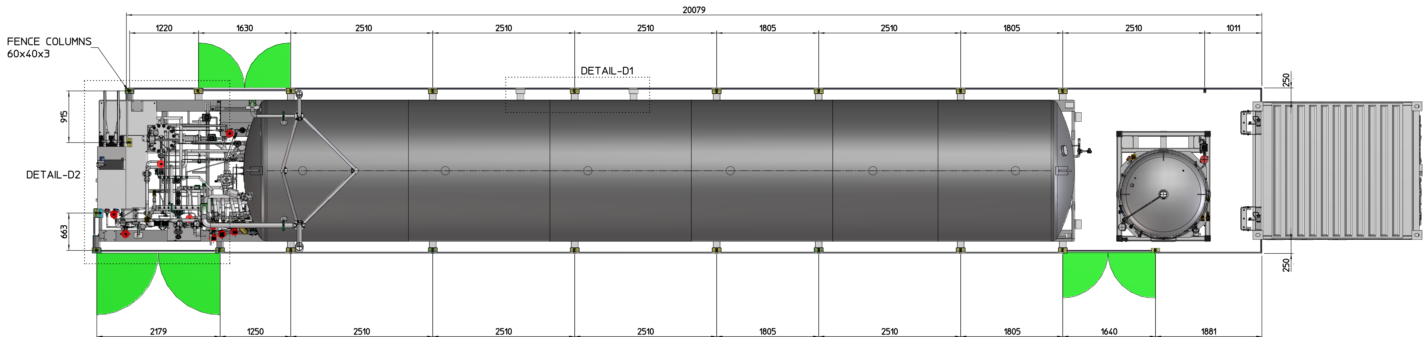
VISTA DALL'ALTO - top view1 SCALE 1:40
