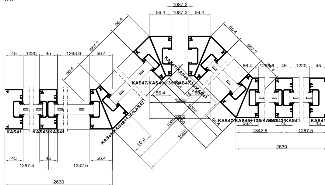
B-B
