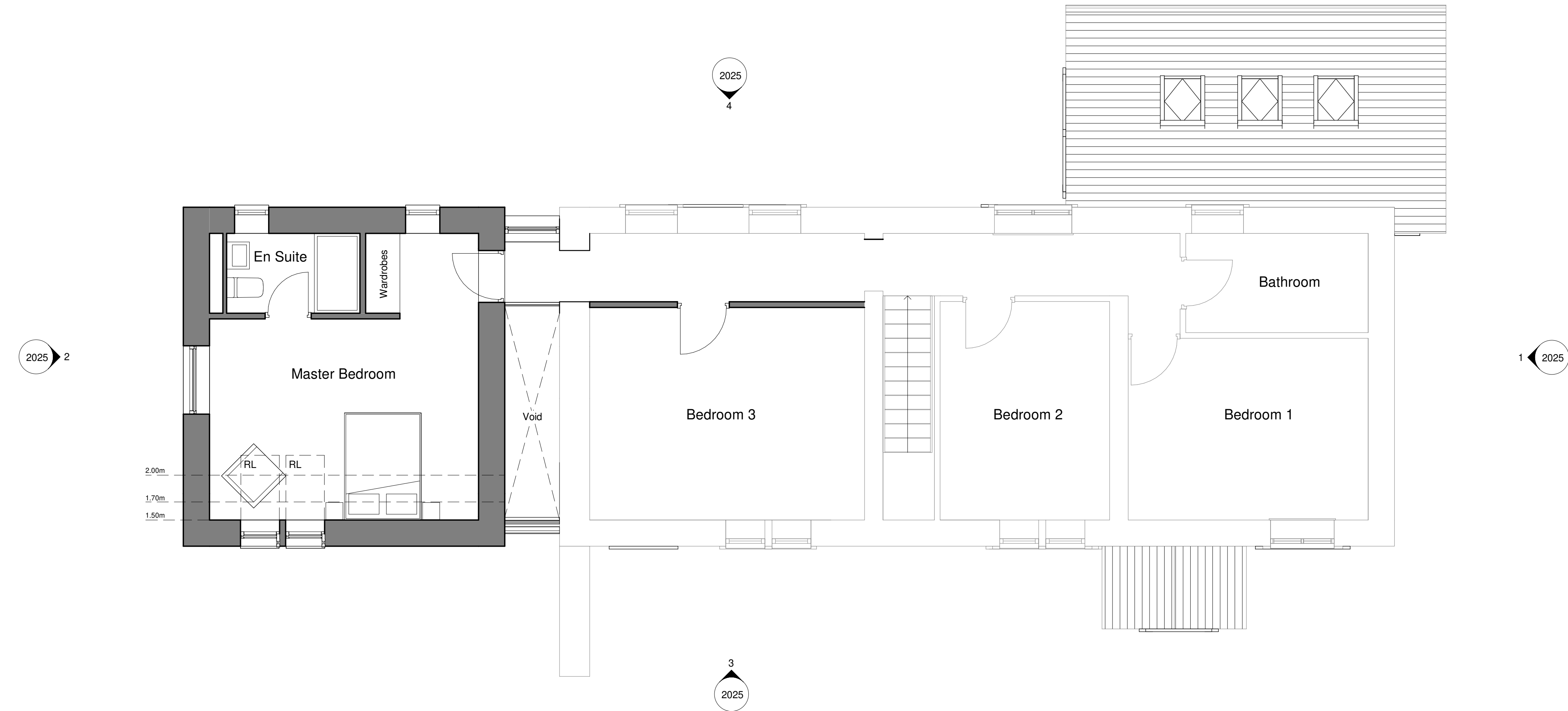
2 | Pro Level 1 1 : 50
