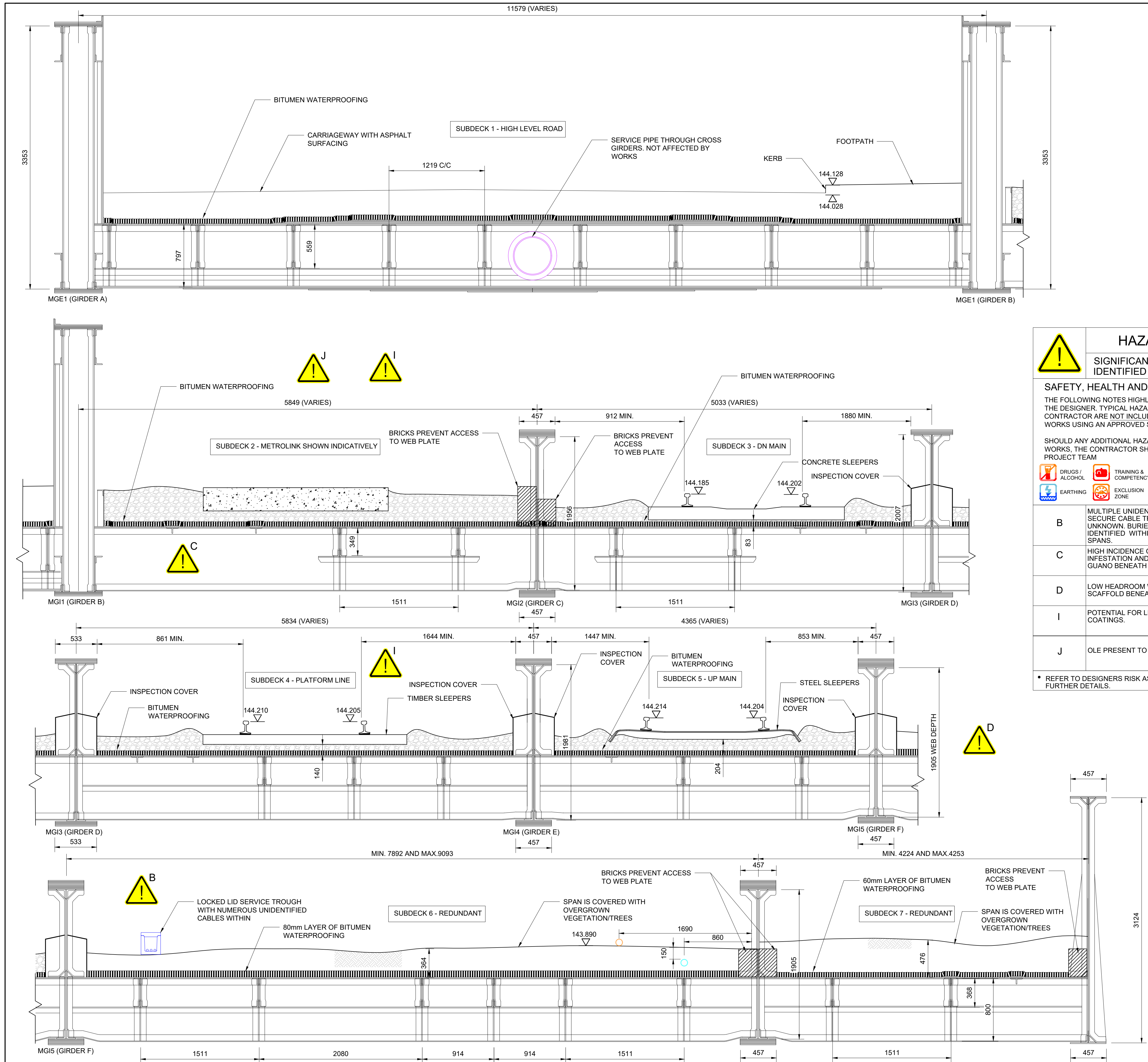
A SECTION 000005 SCALE: 1:25
