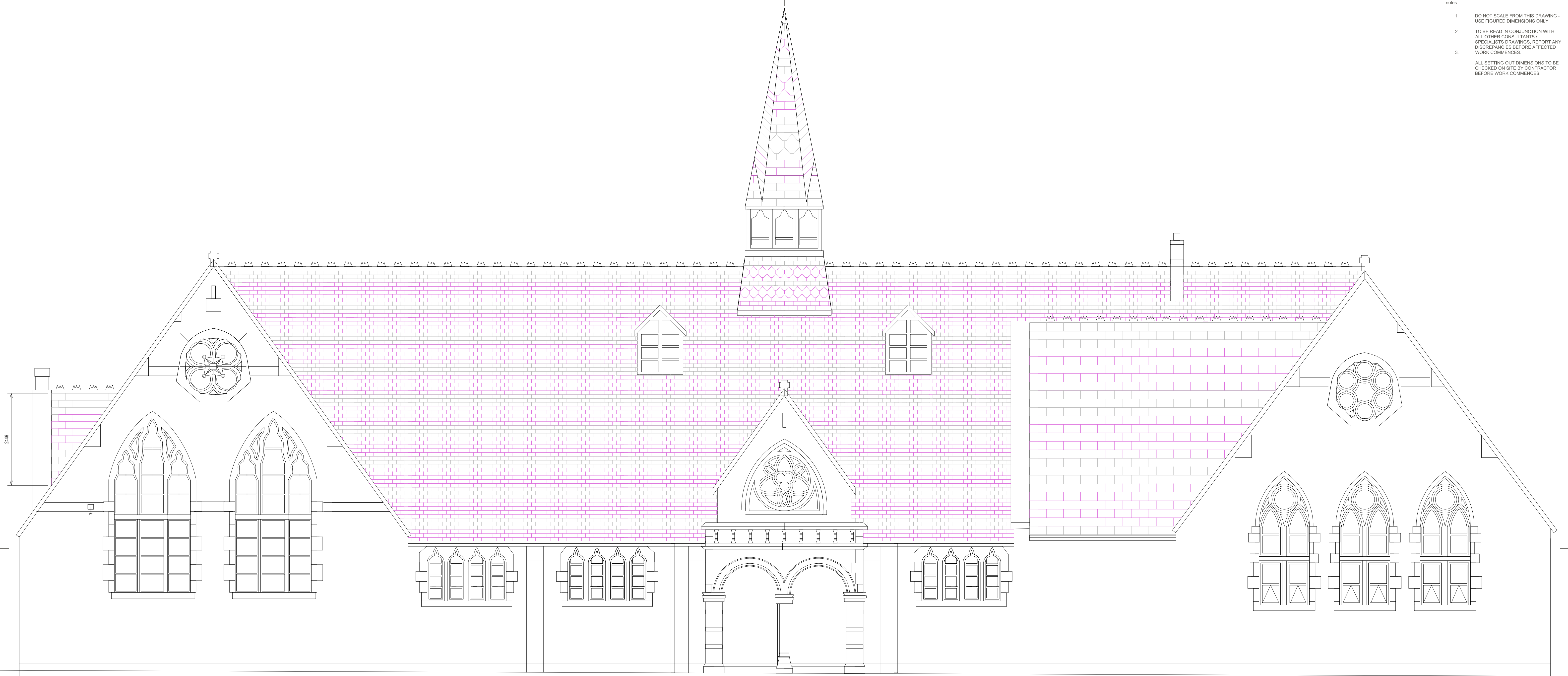
Elevation DD
