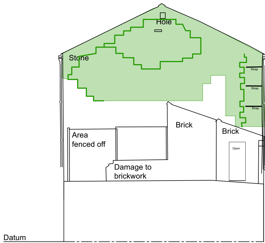
Elevation E
