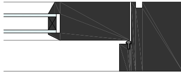
Jamb: Inward Opening Door
