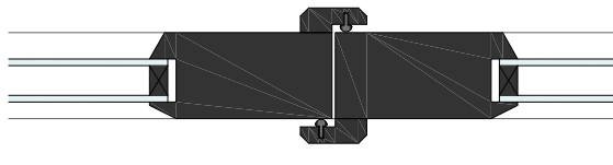
Double Door Stiles
