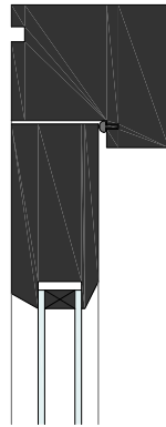
Head: Inward Opening Door
