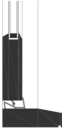
Sill: Inward Opening Door
