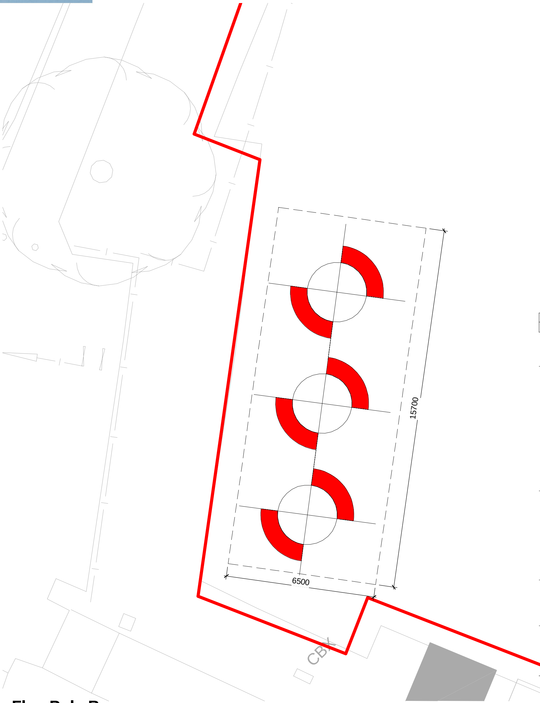
Flag Pole Base 1 : 100
