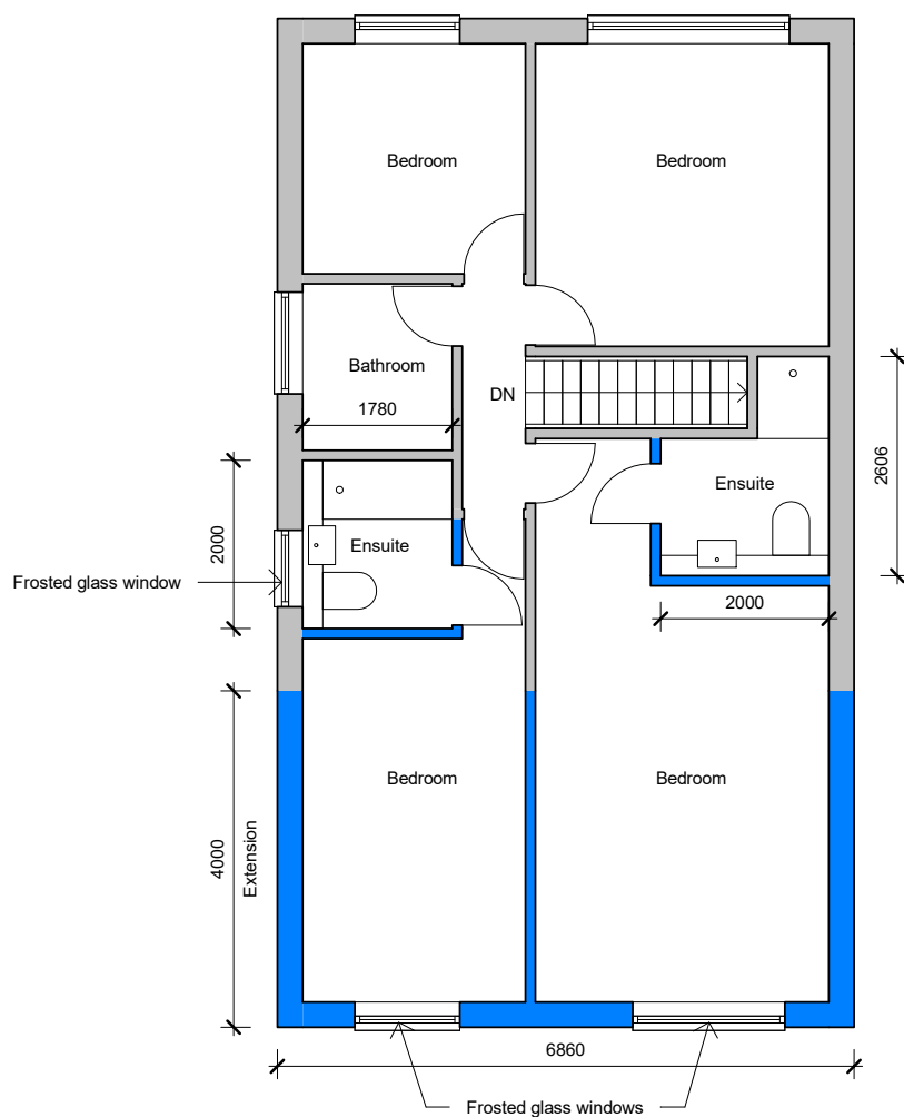
2 Level 1 1 : 100
