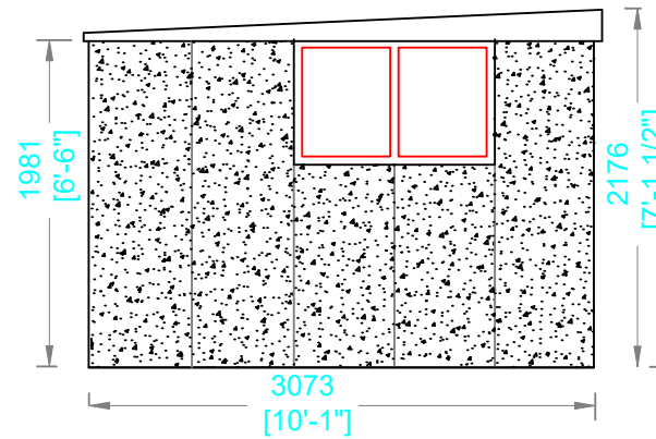
LH ELEVATION
