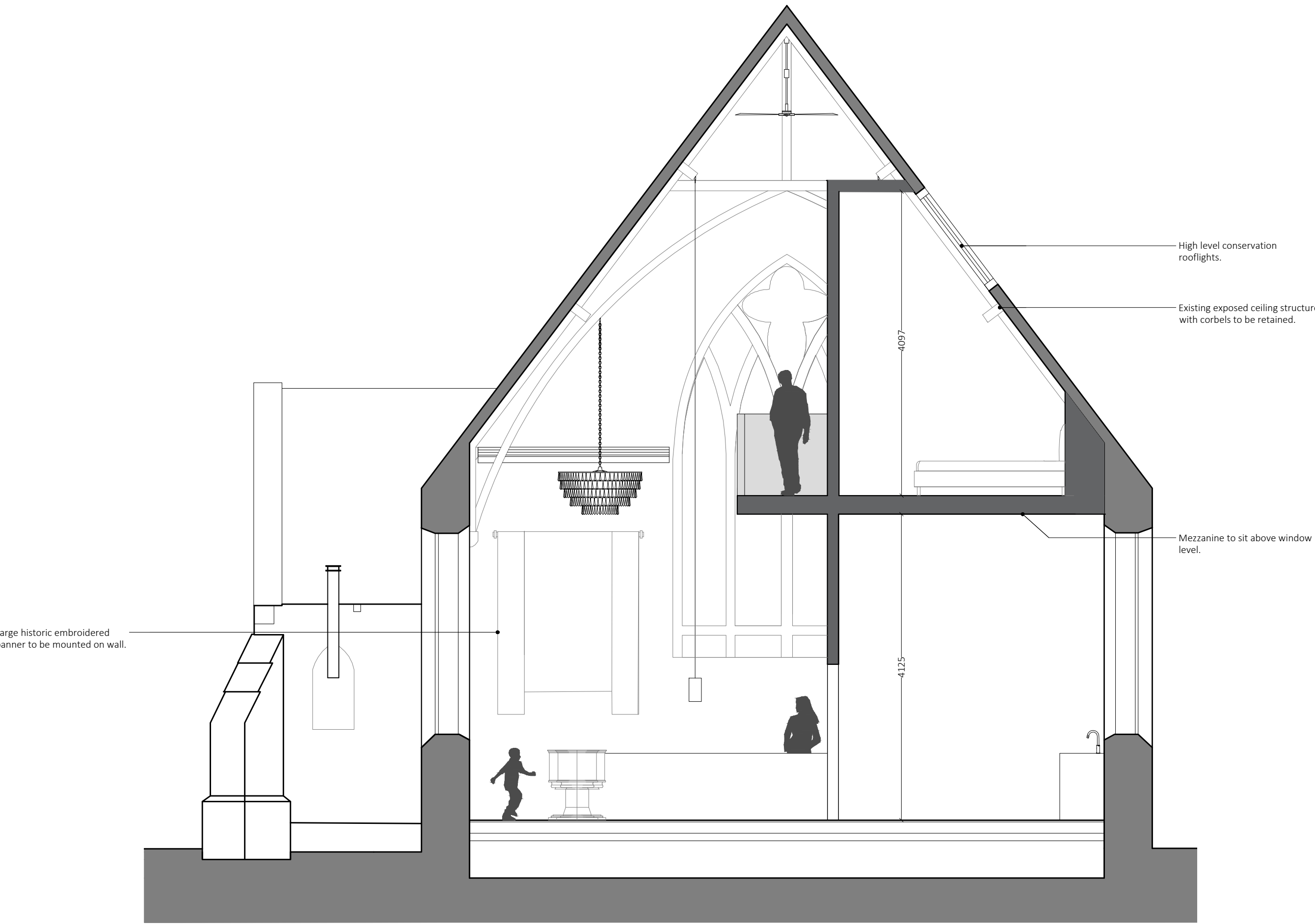
Section A-A
