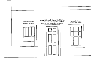
Right Elevation
