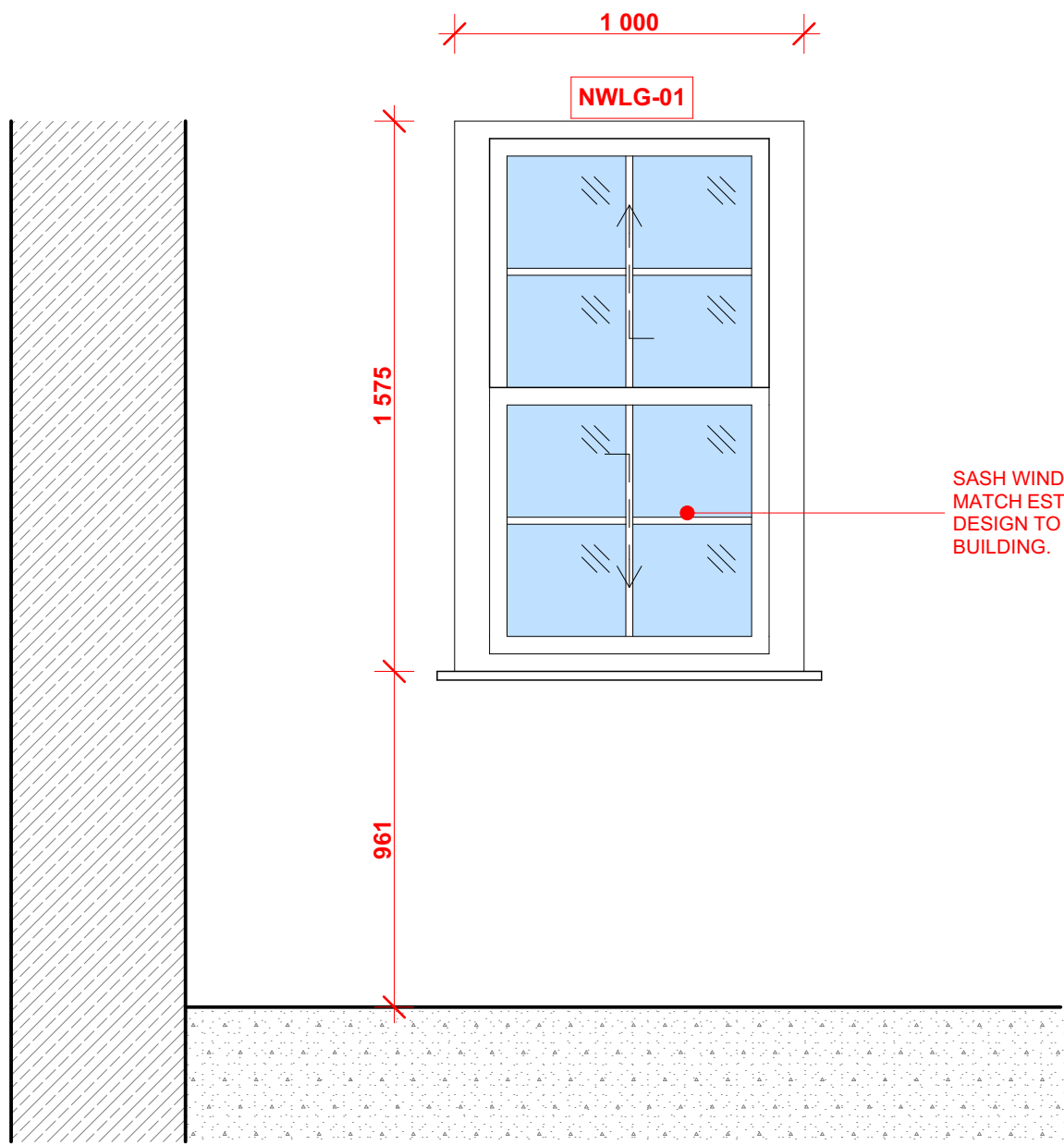
(NWLG-01) ELEVATION VIEW SCALE: 1:20
