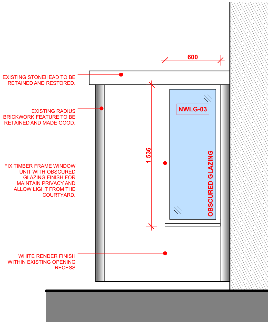
(NWLG-03) ELEVATION VIEW SCALE: 1:20
