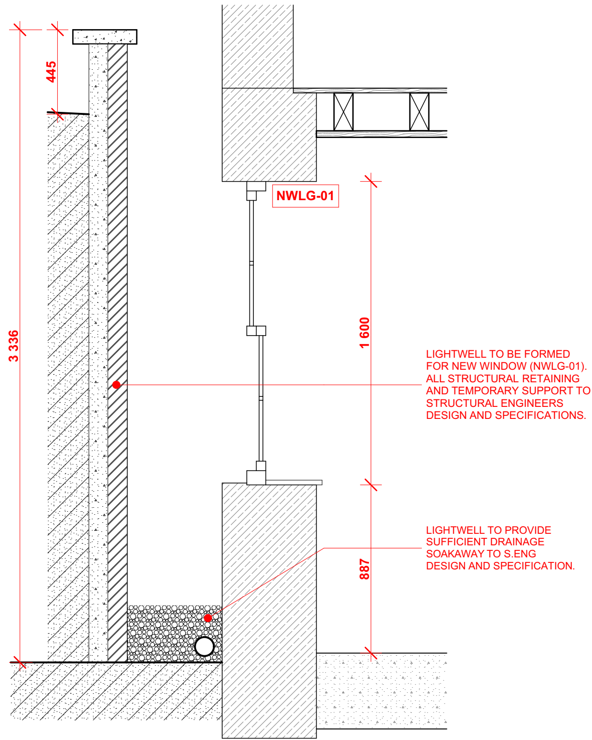
(NWLG-01) SECTION VIEW SCALE: 1:20
