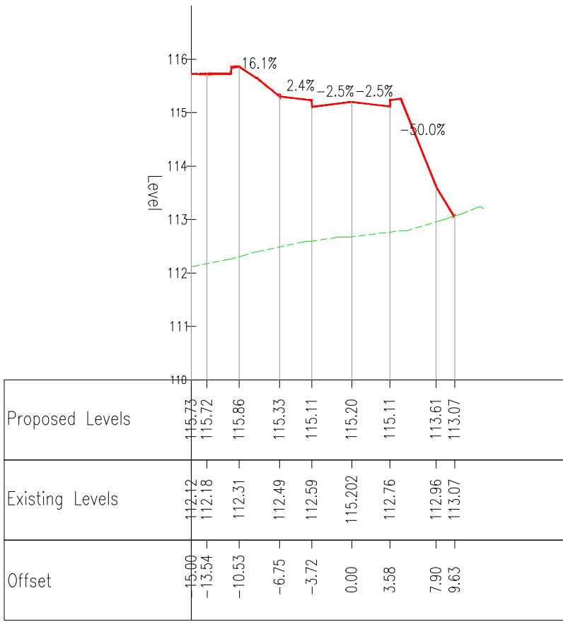
Chainage 70.000
