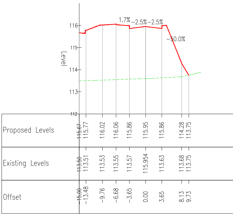
Chainage 90.000
