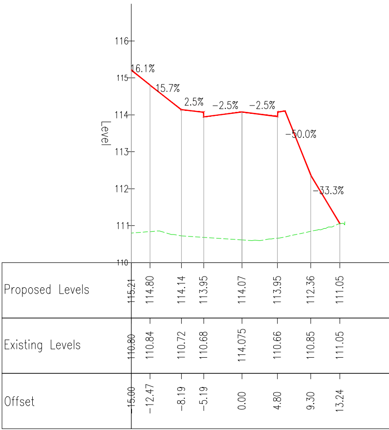
Chainage 40.000
